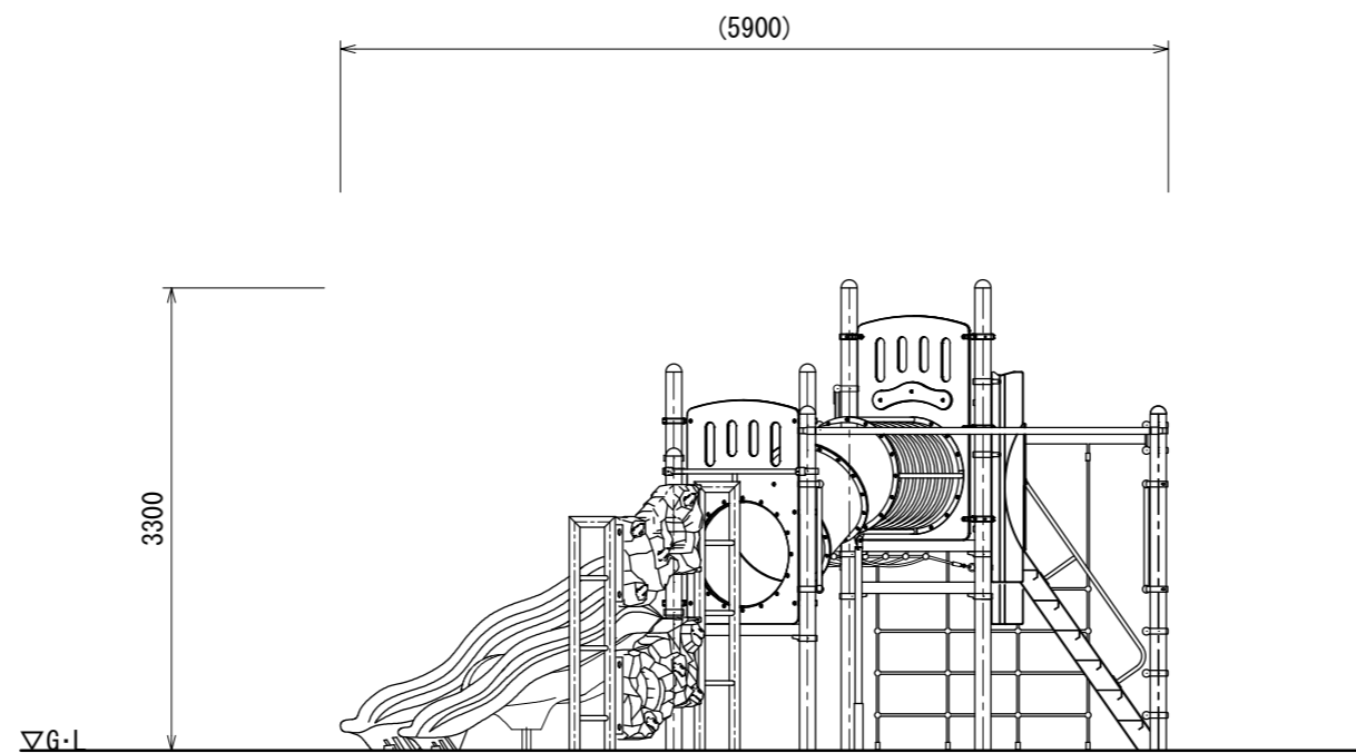
B立面図
