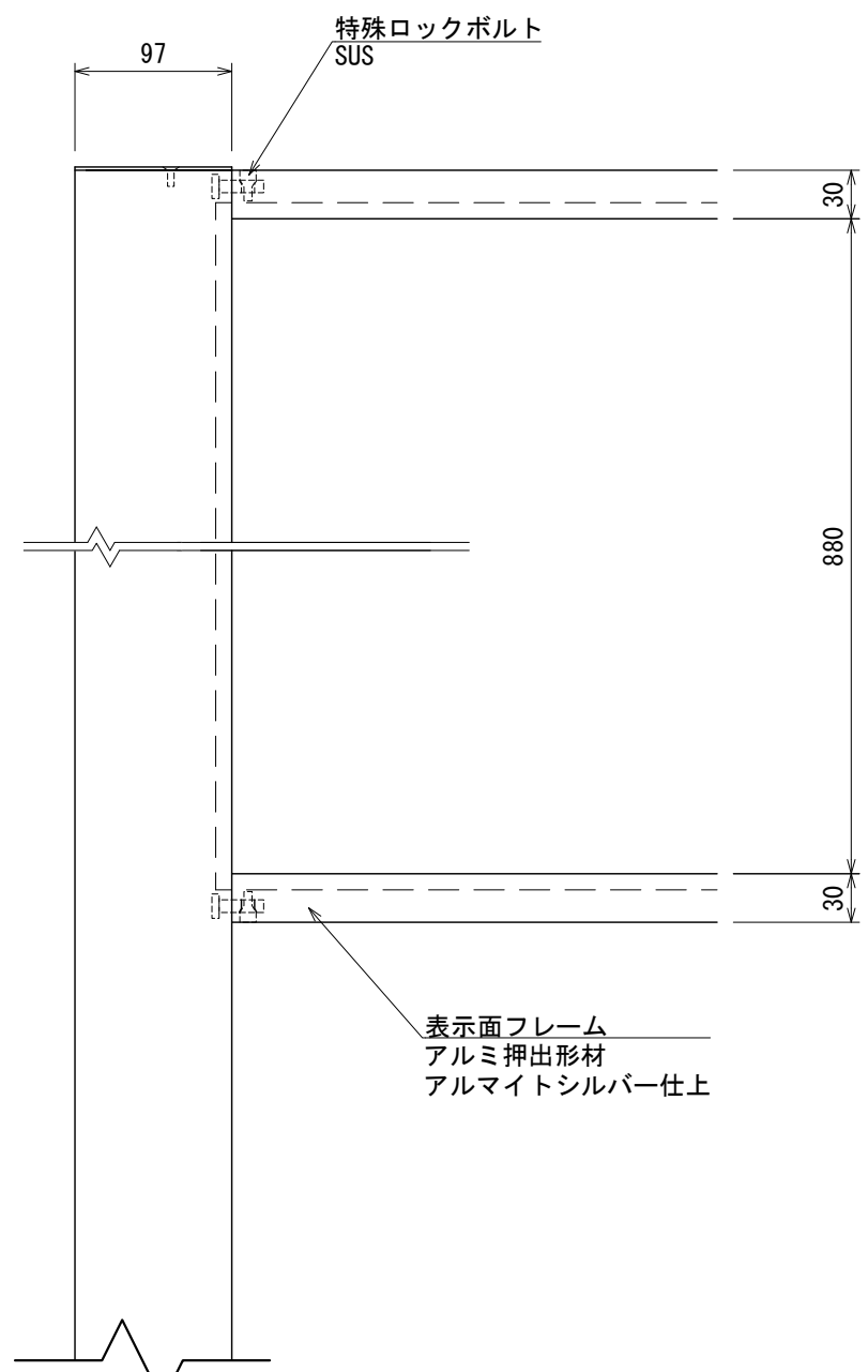
【正面図 S=1:5】
