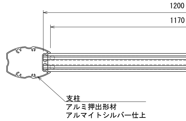
【平面図 S=1:5】
