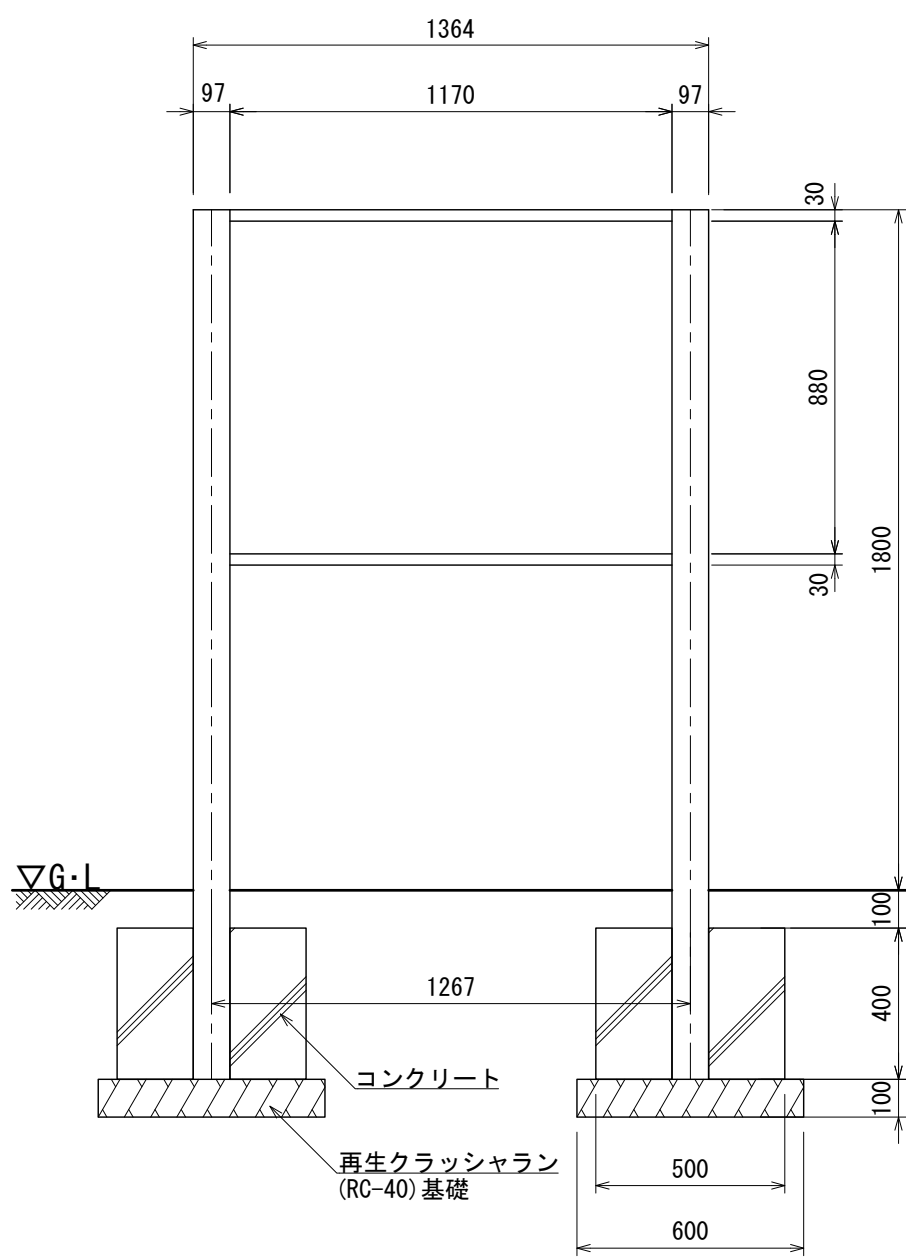
【正面図】
