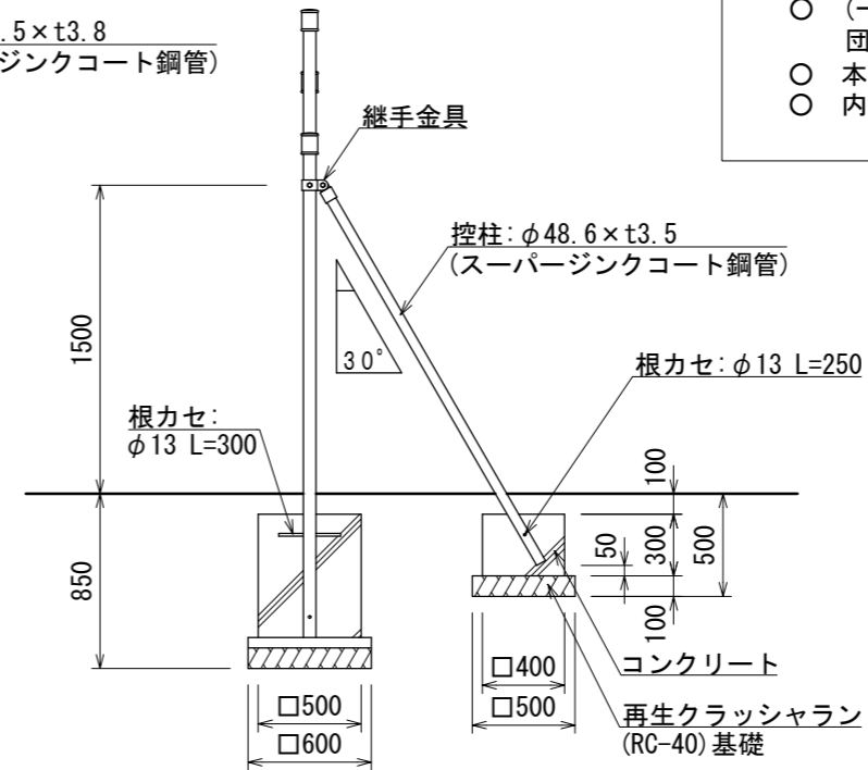
側面図
