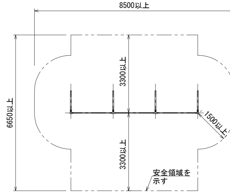
安全領域図 S=1:100
