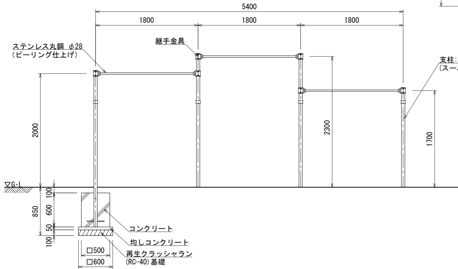
立面図
