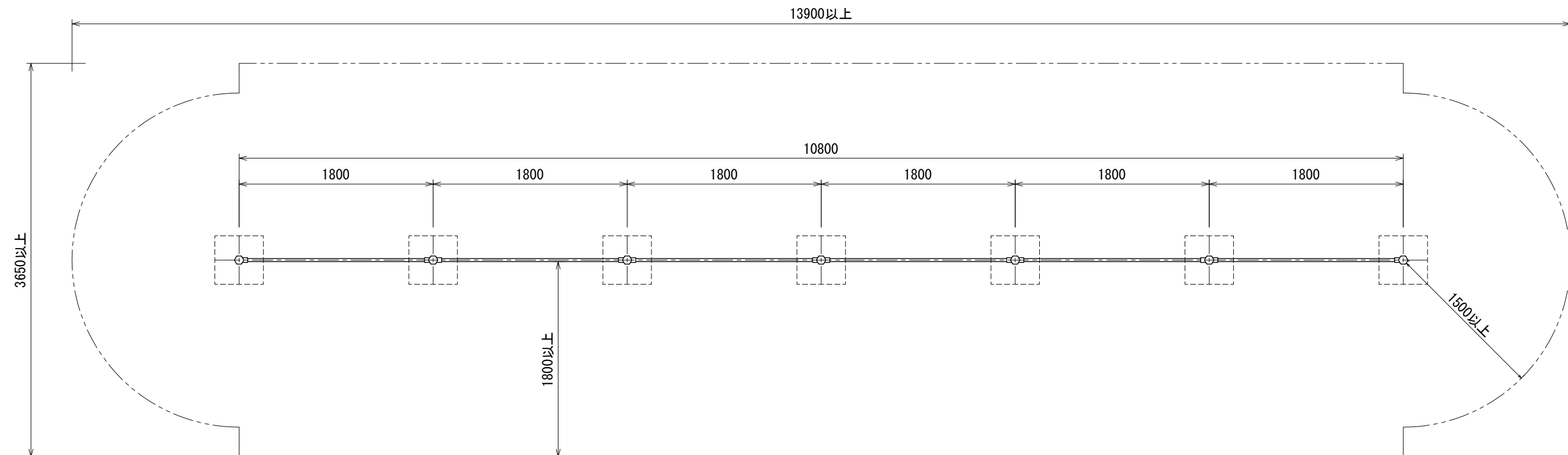
平面図
