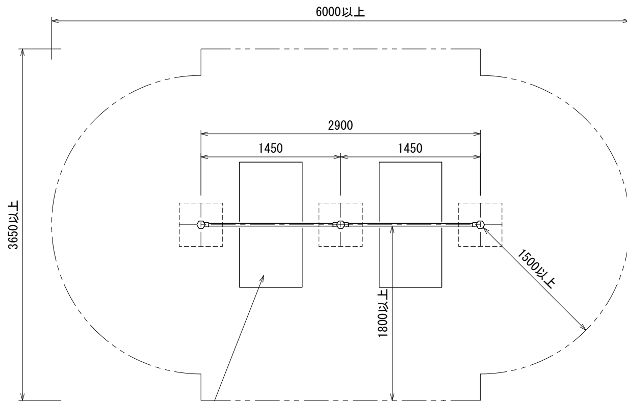
平面図
