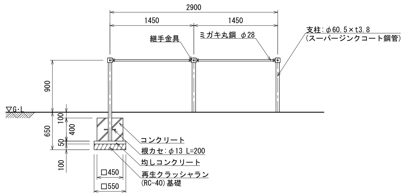
立面図
