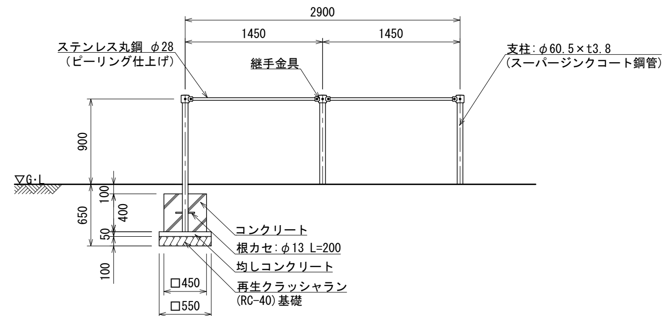
立面図
