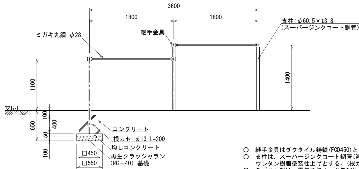
立面図
