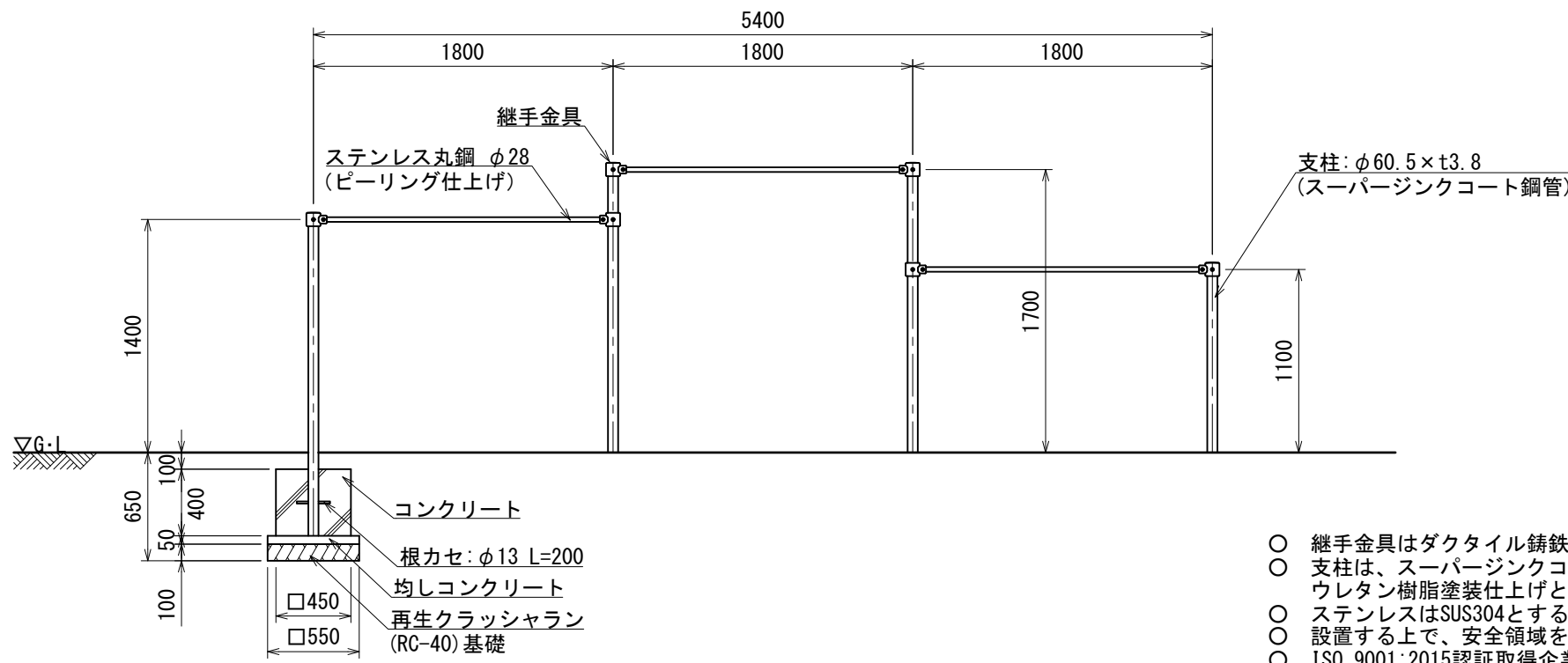
立面図
