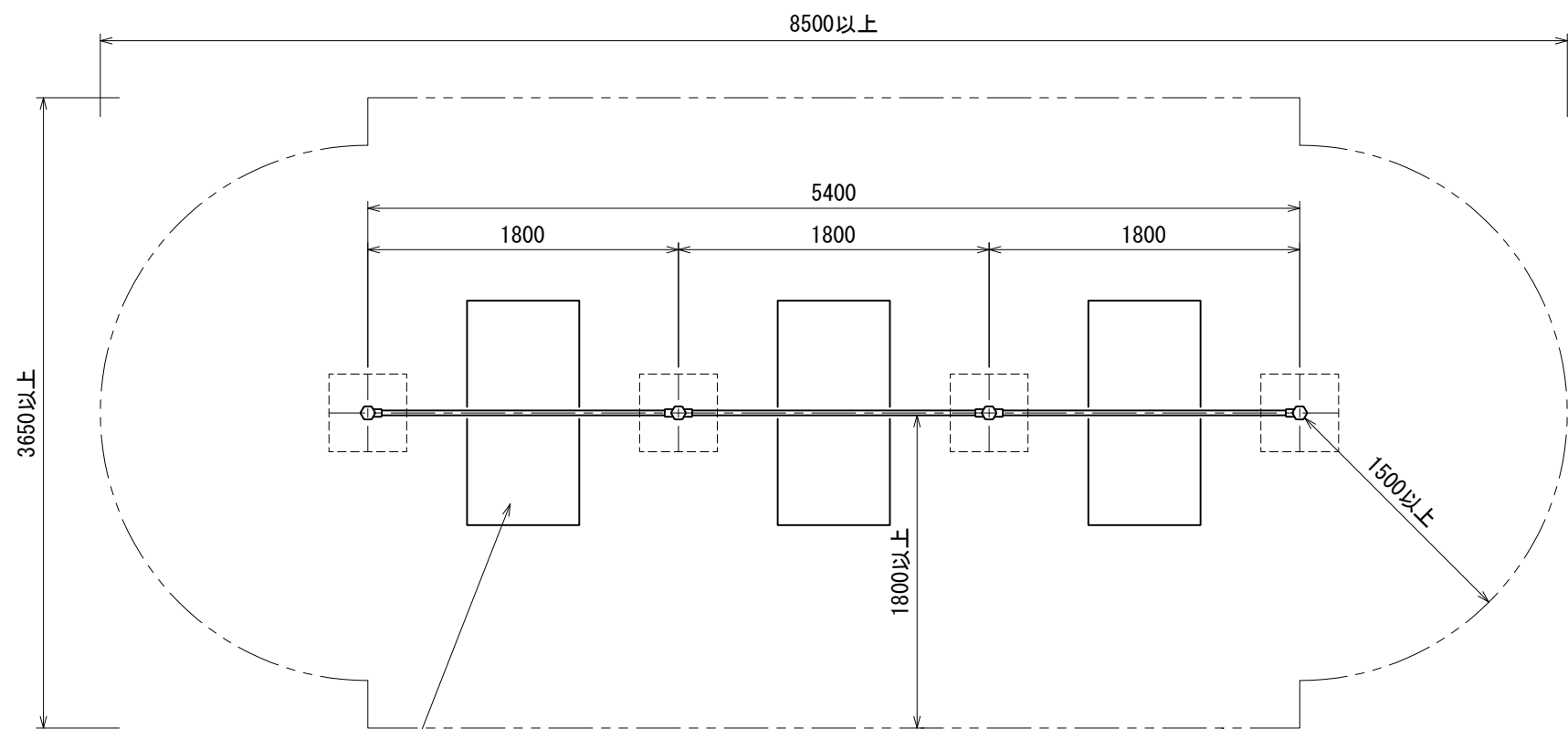
平面図
