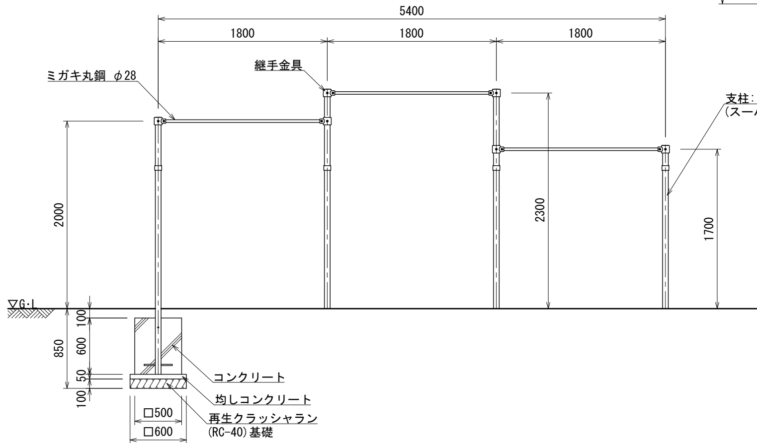
立面図
