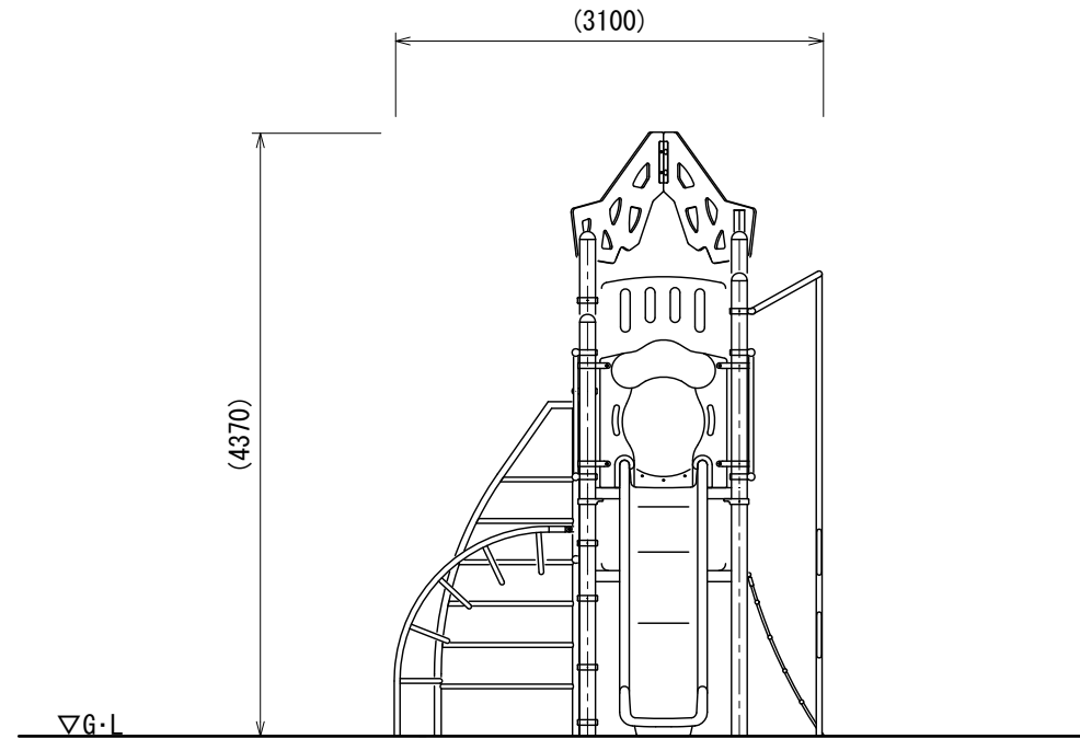
B立面図
