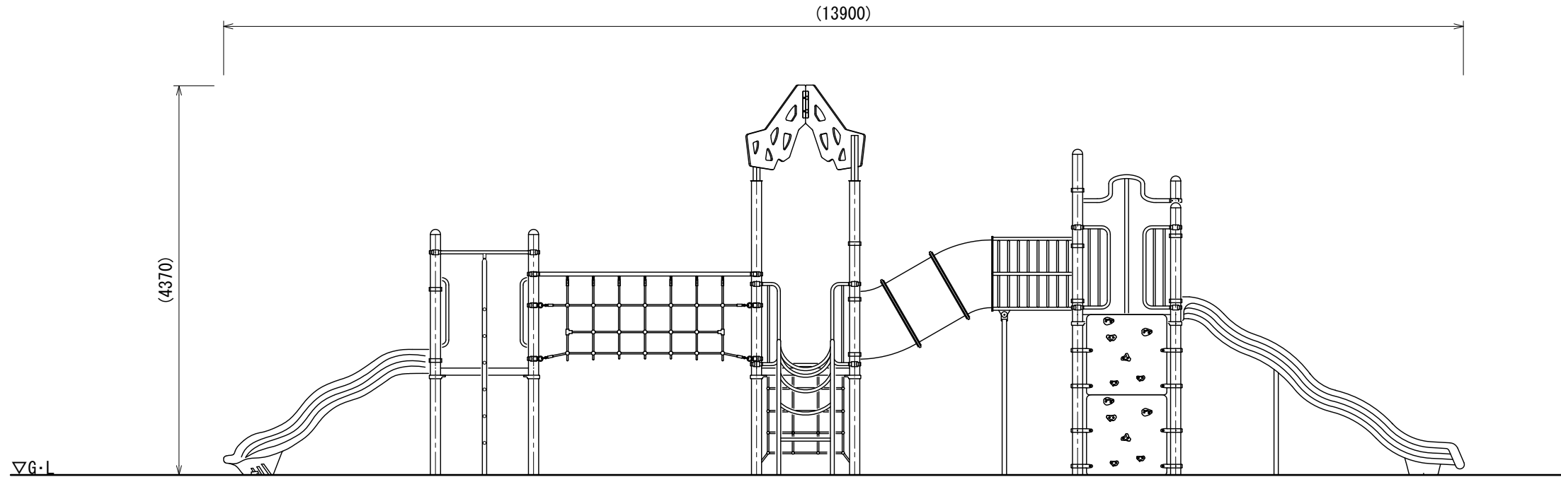
A立面図
