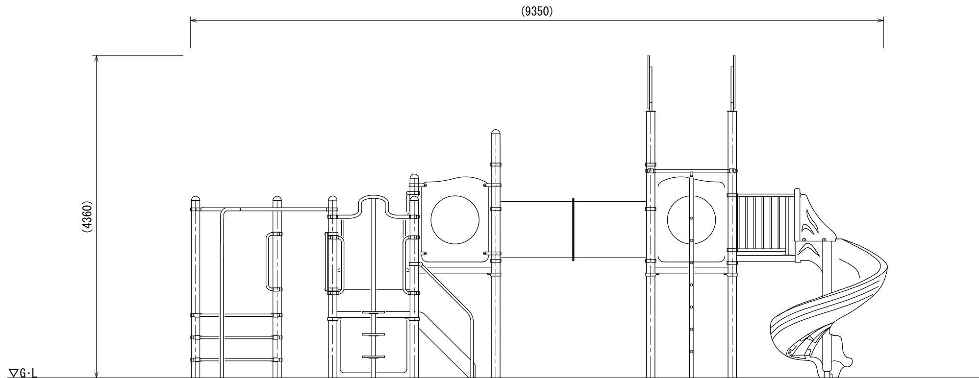
A立面図
