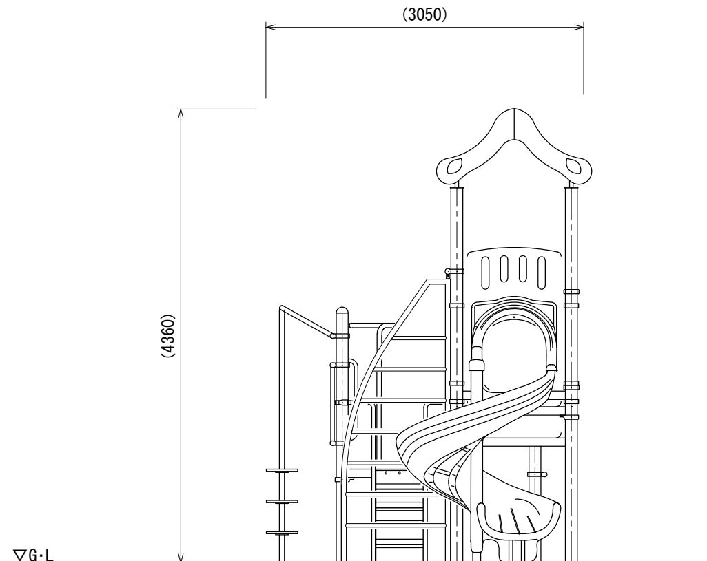
B立面図
