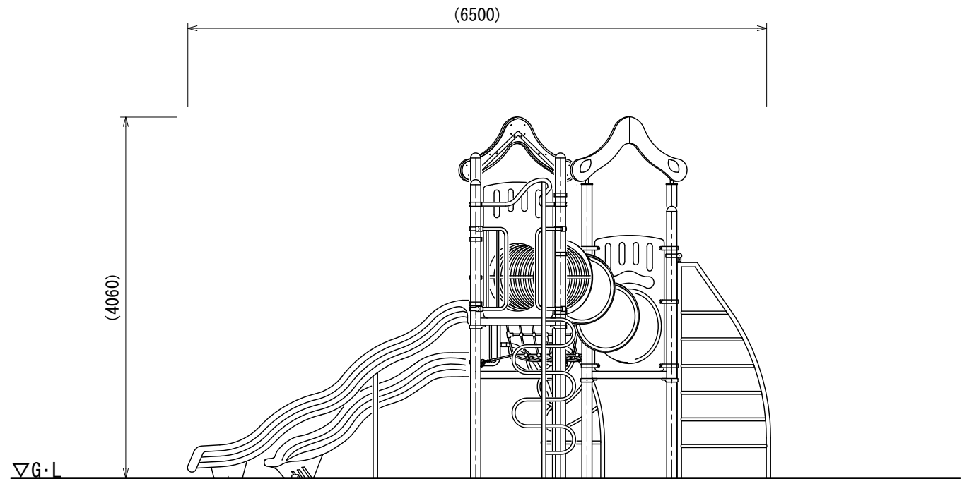
B立面図
