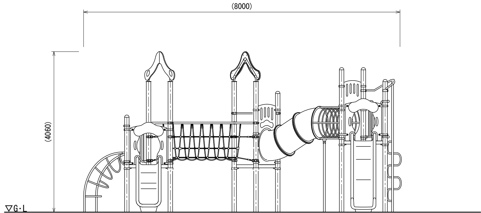
A立面図
