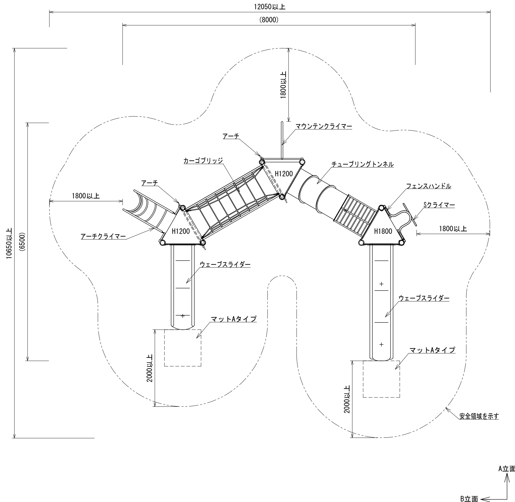
平面図
