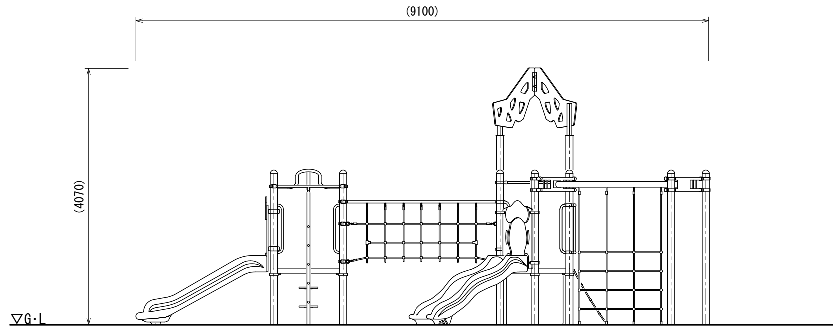
A立面図
