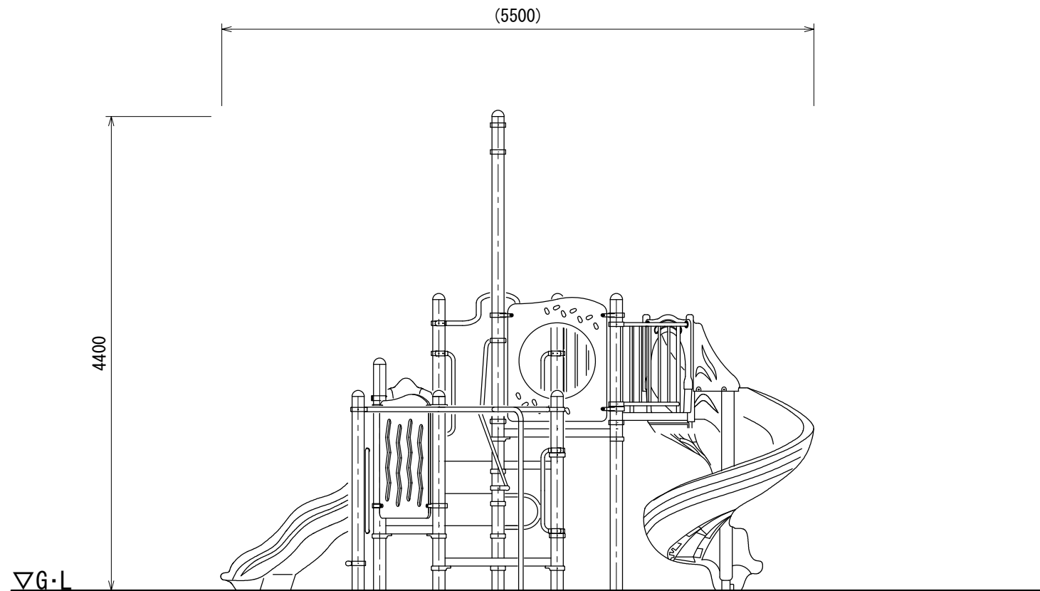
B立面図
