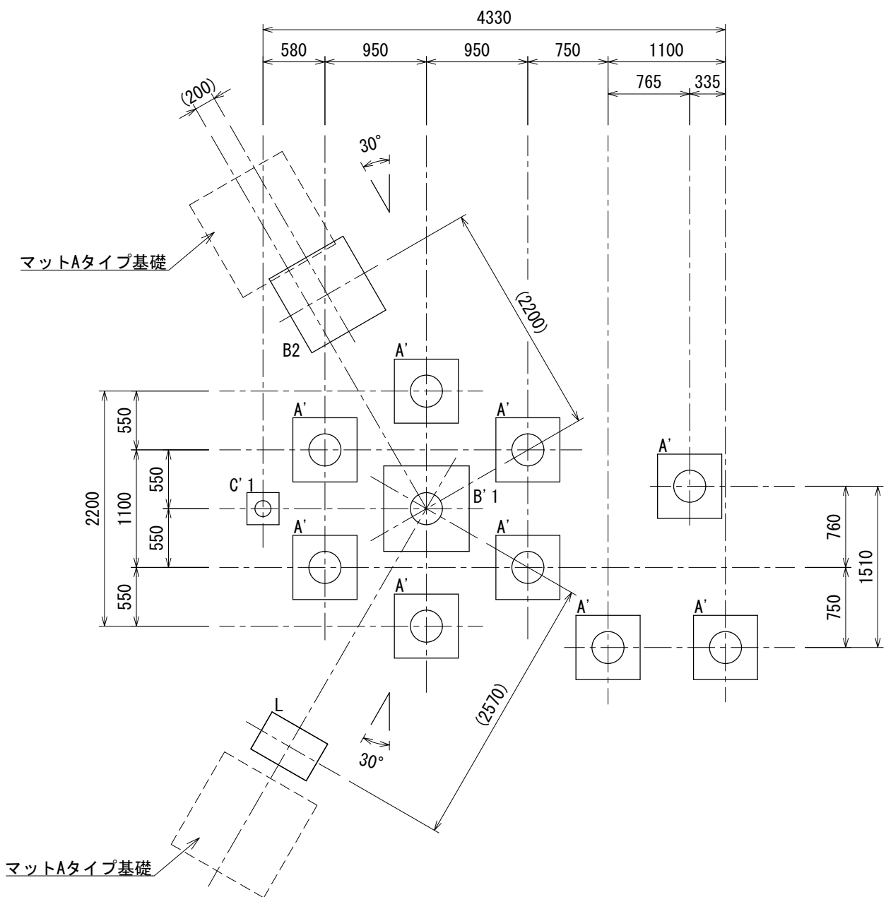
基礎伏図
