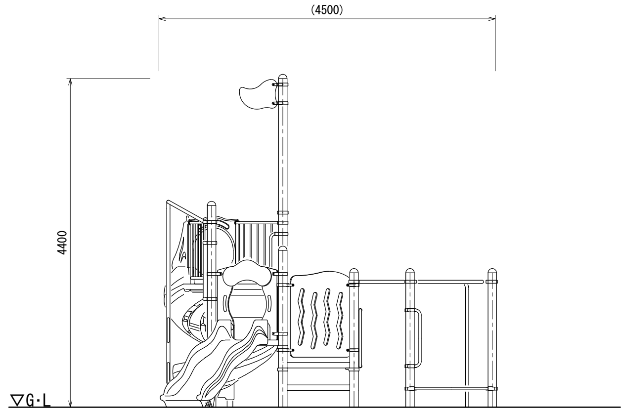
A立面図
