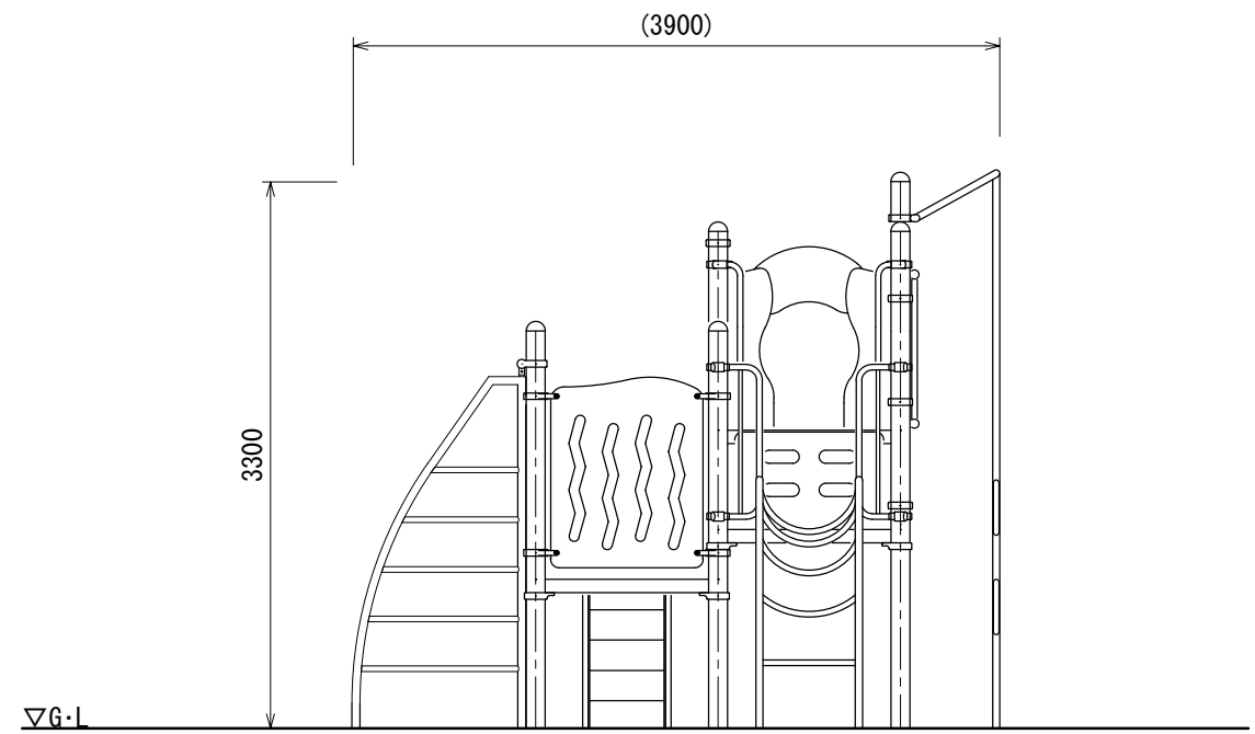
B立面図
