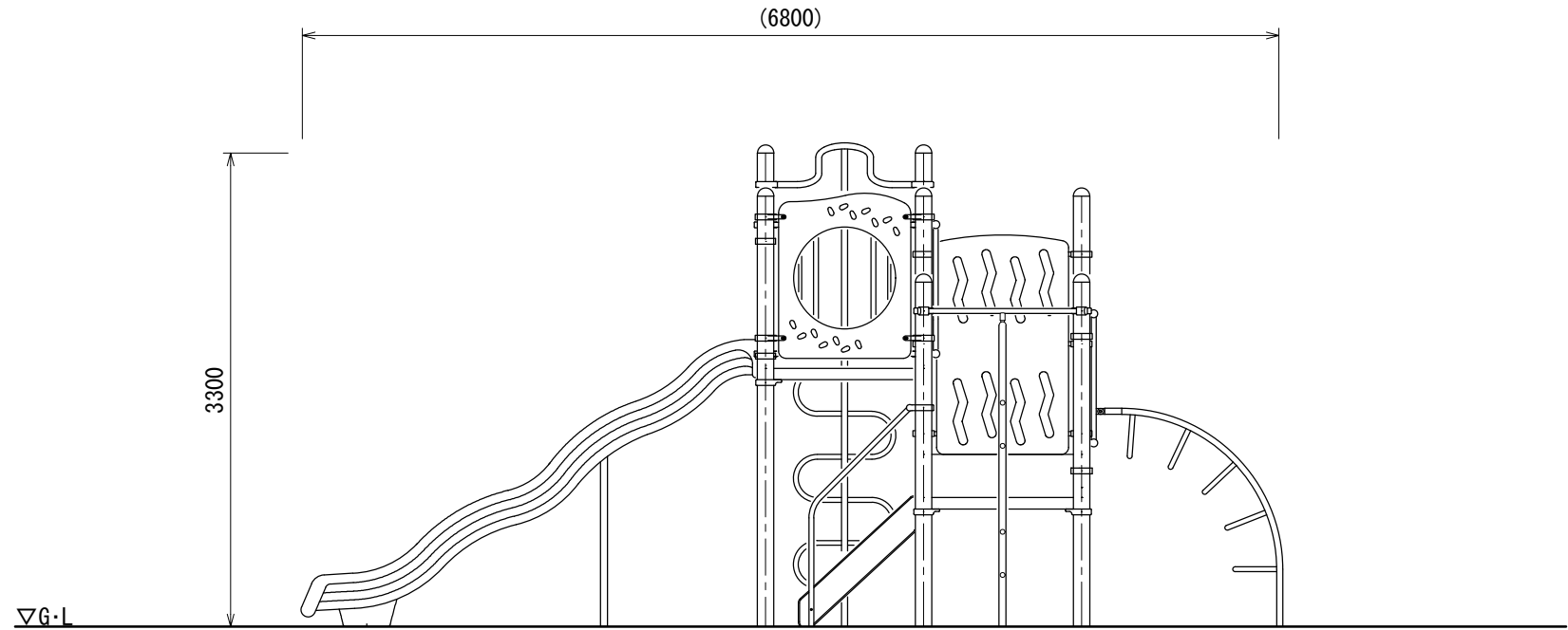
A立面図
