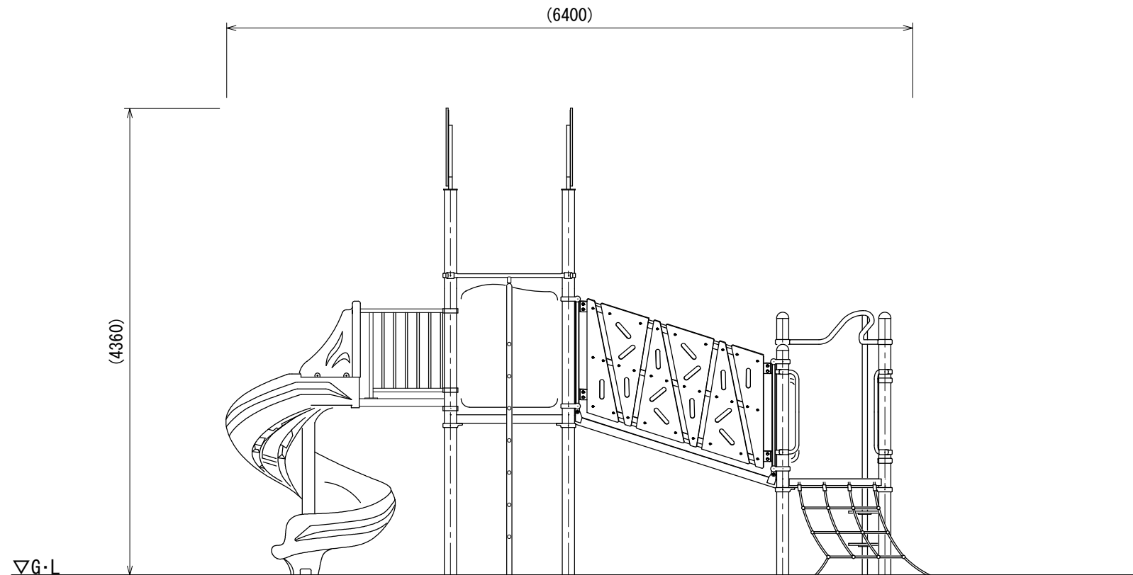
A立面図
