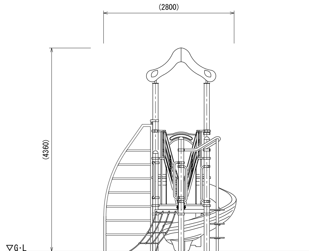
B立面図
