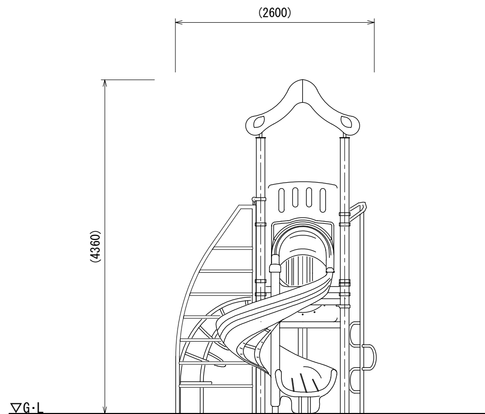
B立面図
