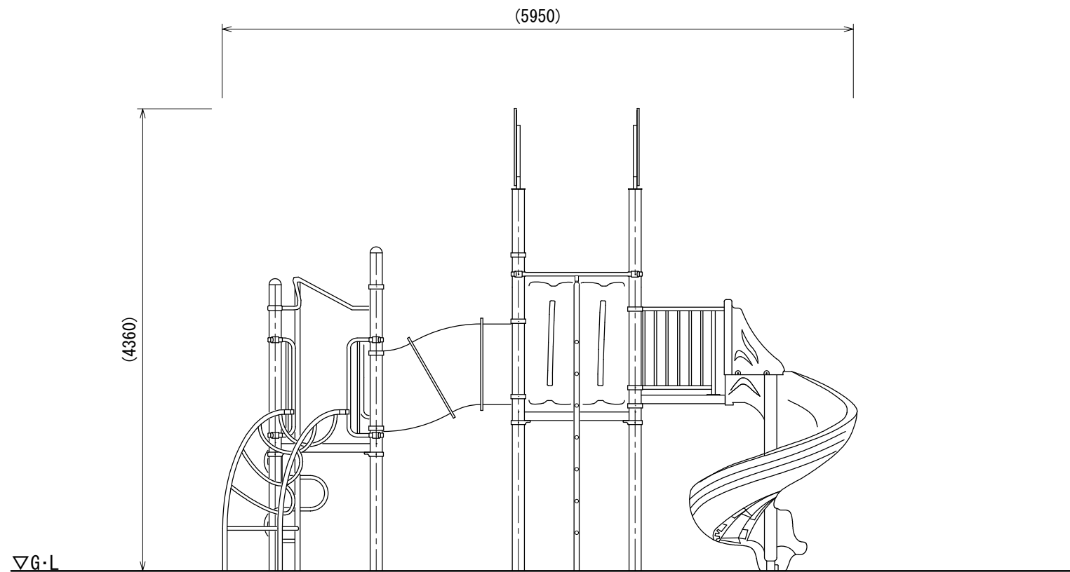
A立面図
