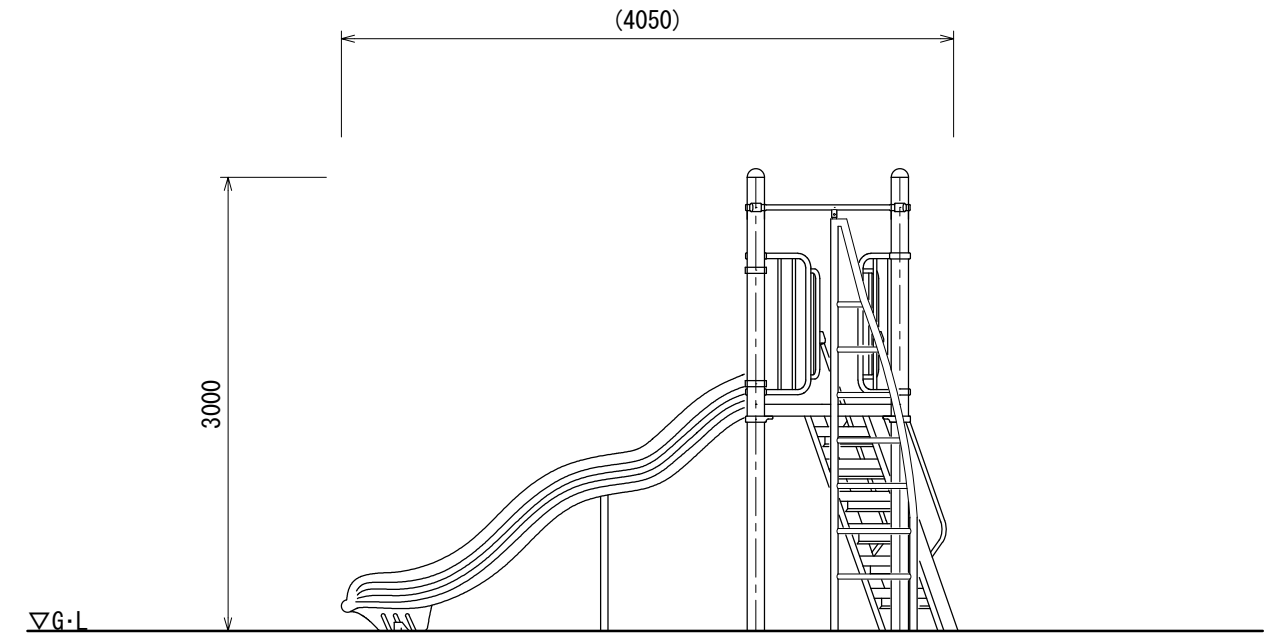
A立面図
