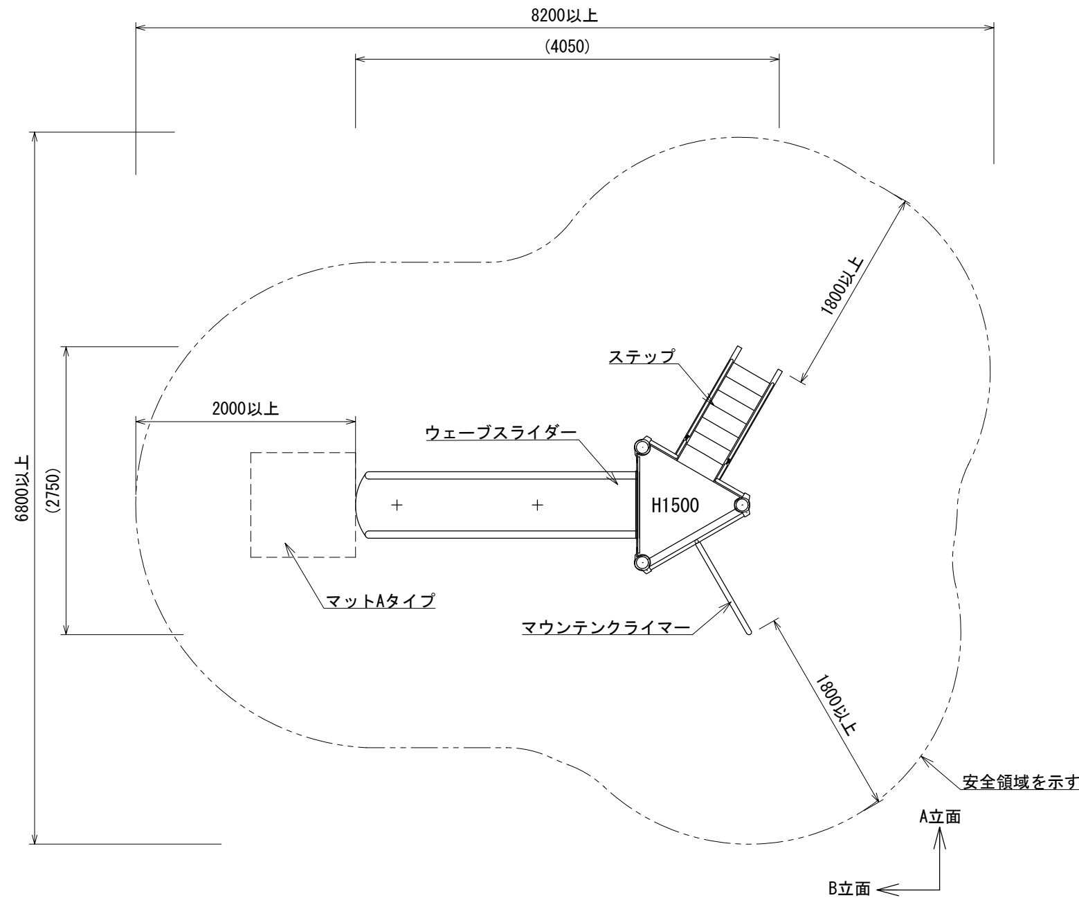
平面図
