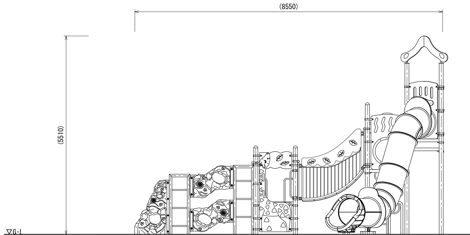
A立面図
