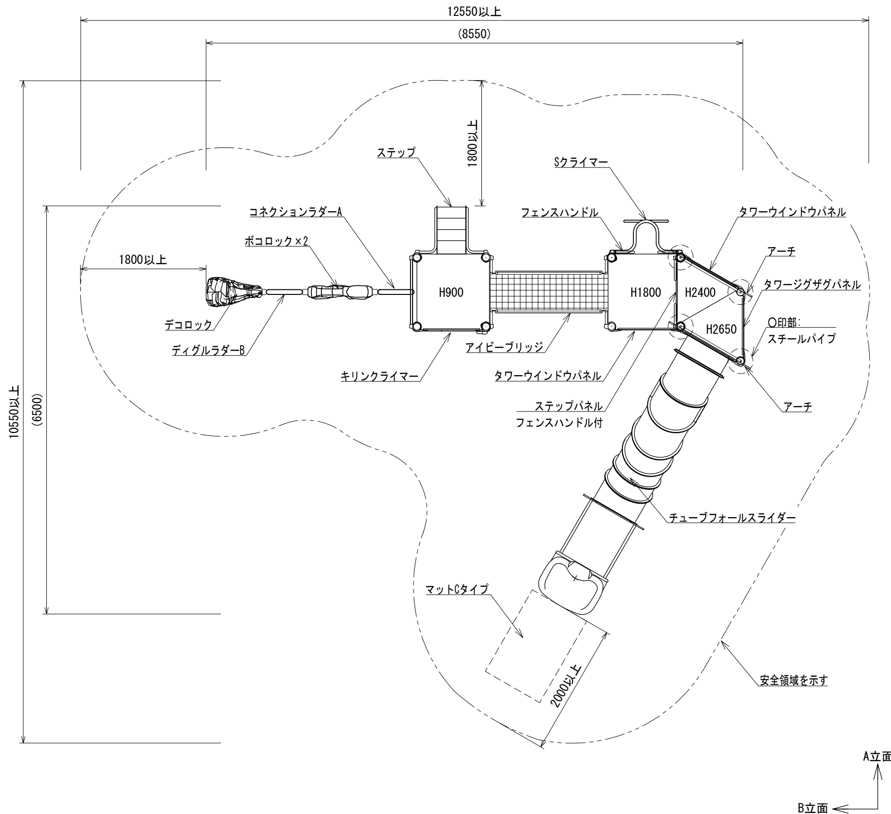
平面図
