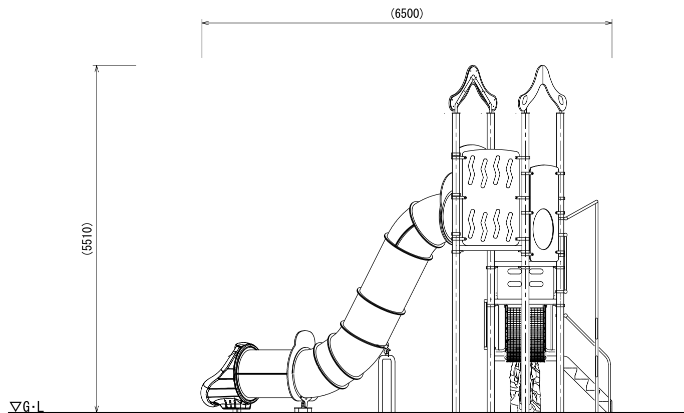
B立面図
