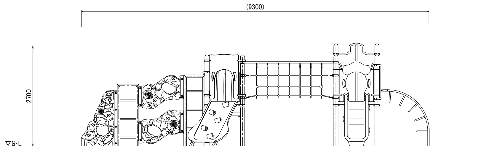
A立面図
