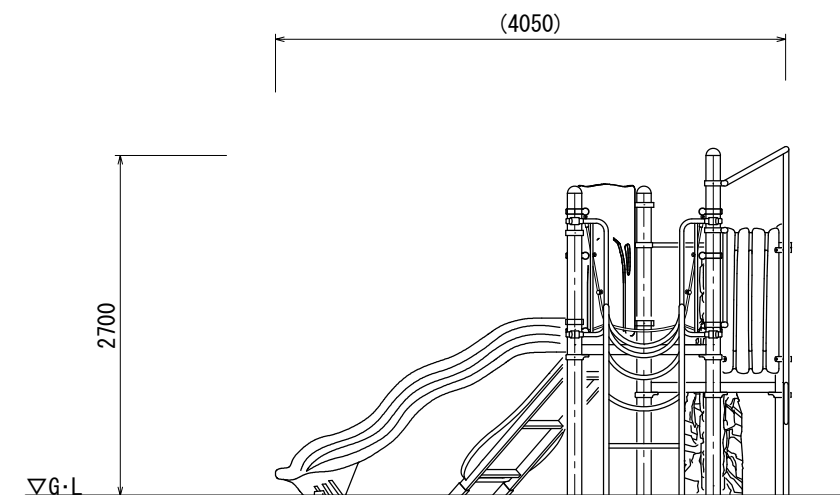
B立面図
