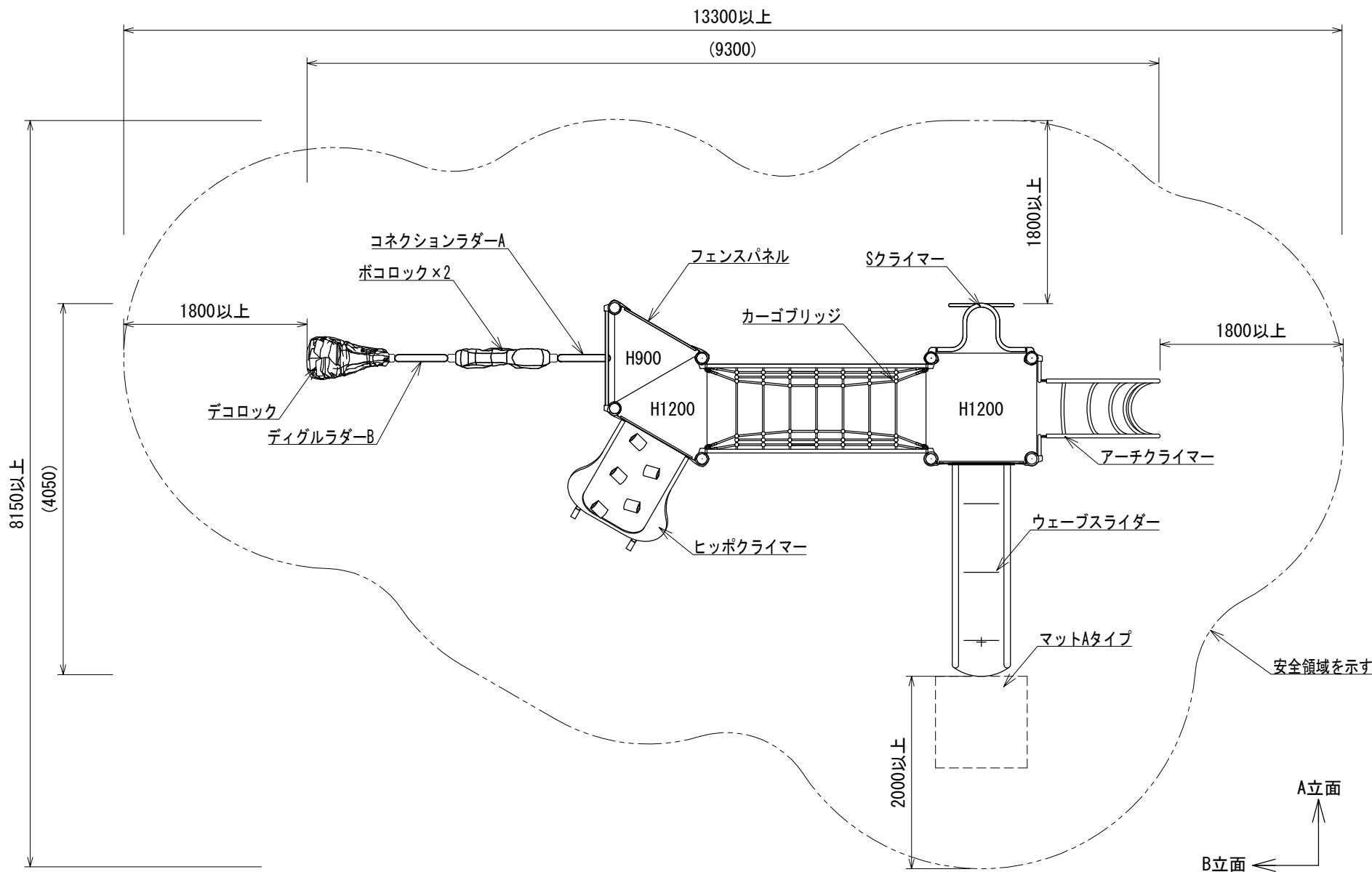
平面図
