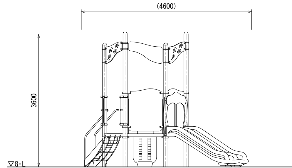
A立面図
