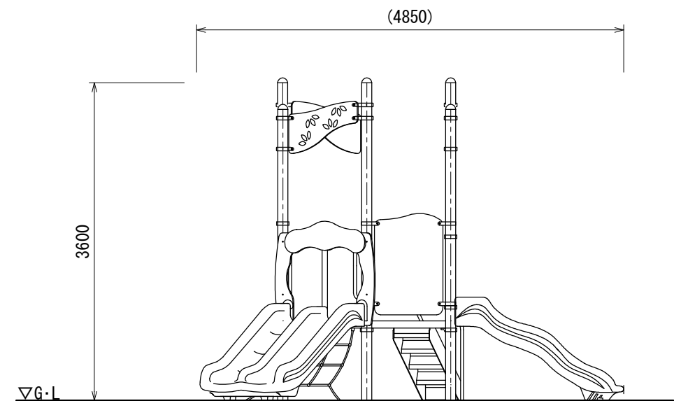
B立面図
