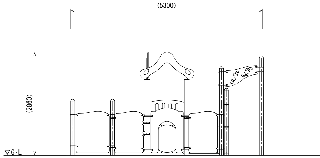
A立面図
