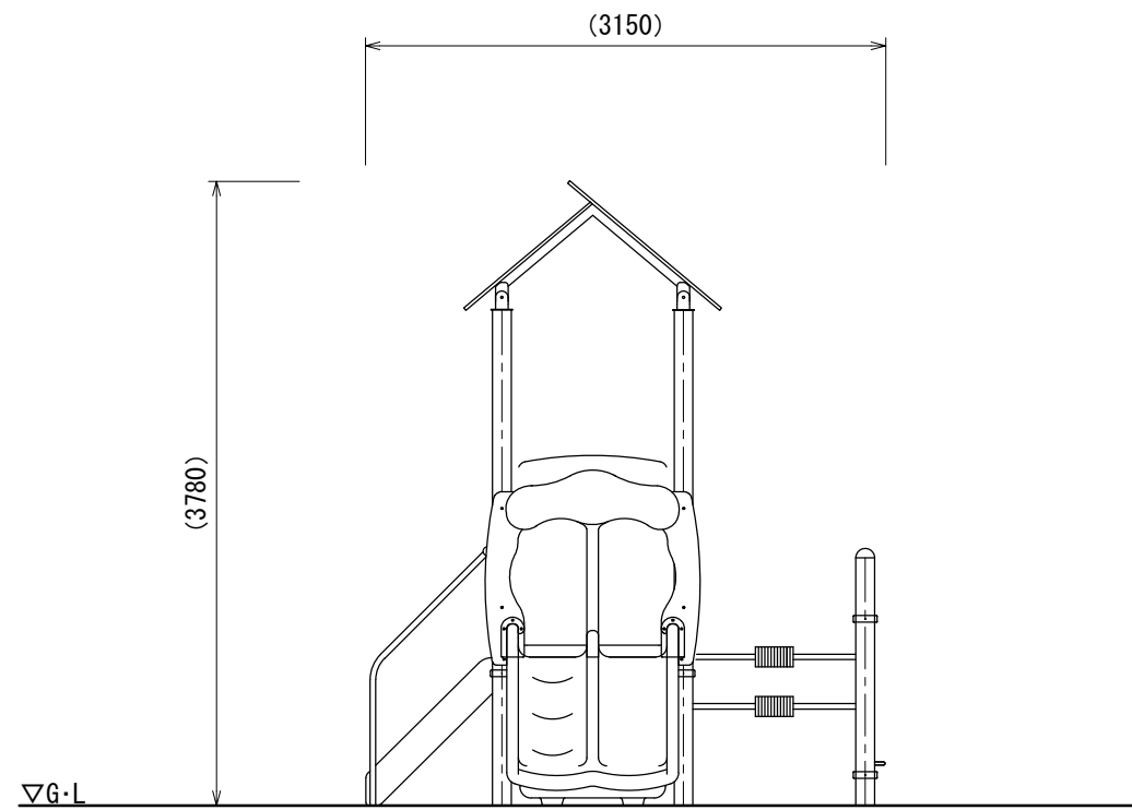
A立面図
