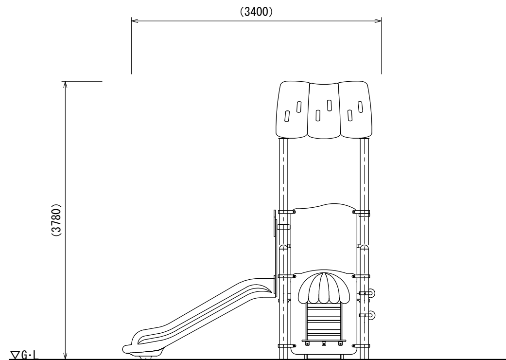
B立面図
