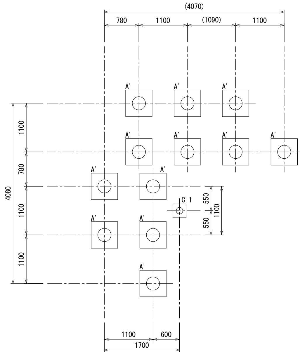
基礎伏図
