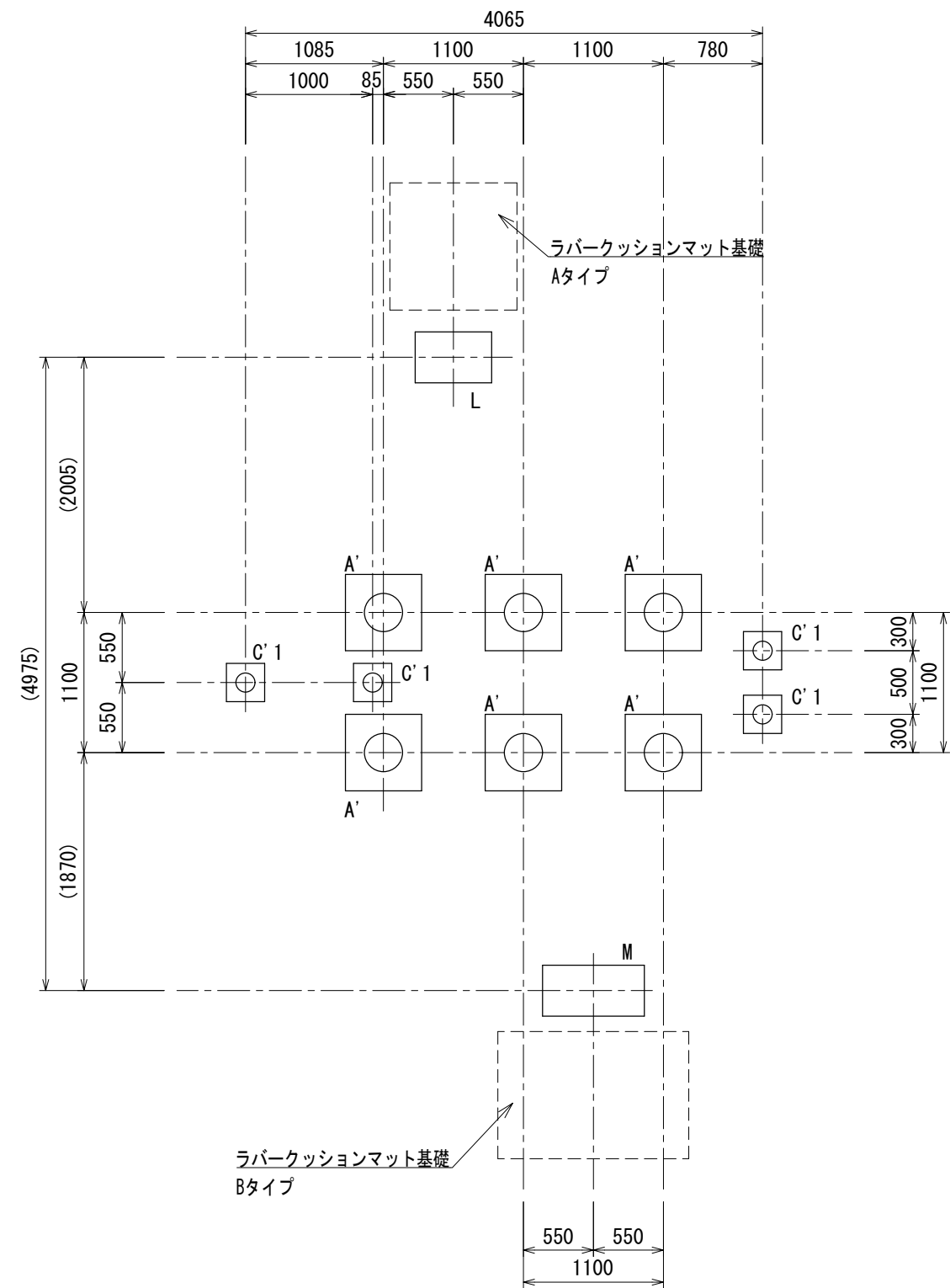
基礎伏図
