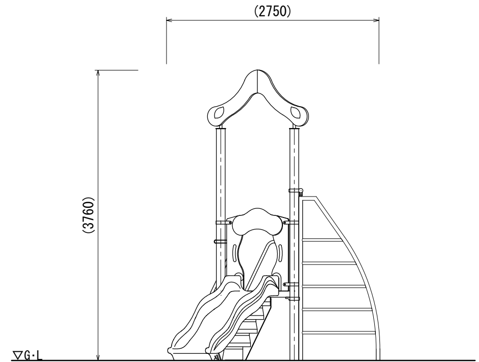
A立面図
