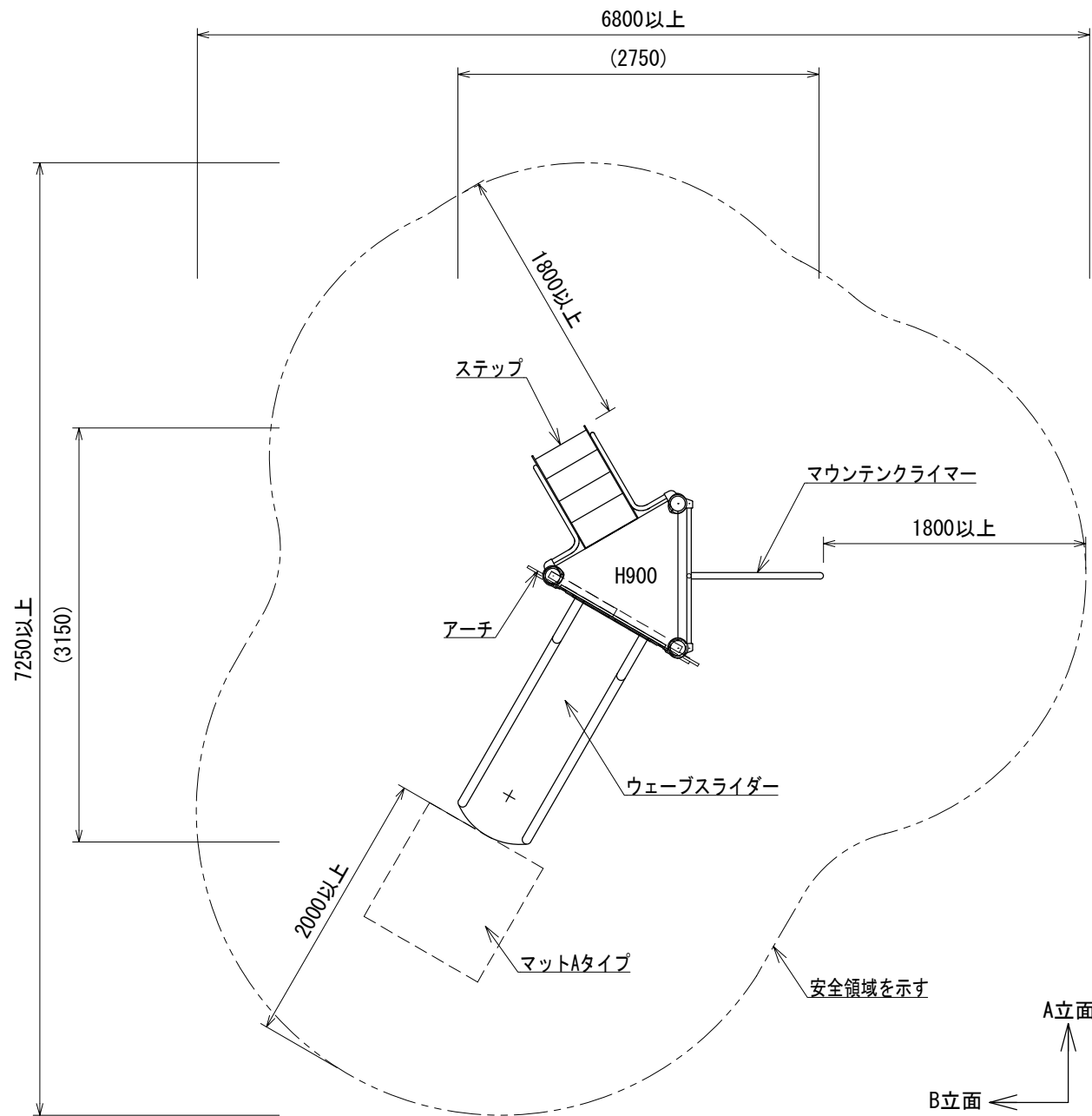
平面図
