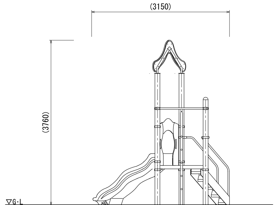
B立面図
