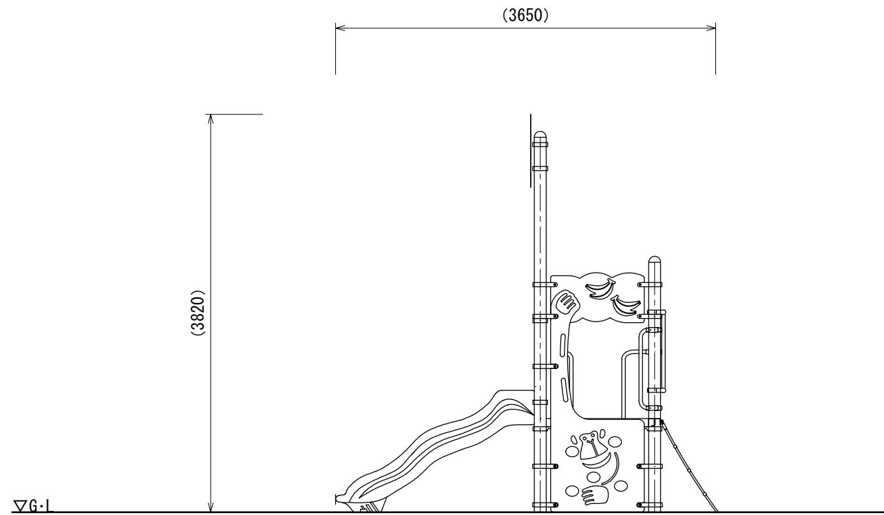
A立面図
