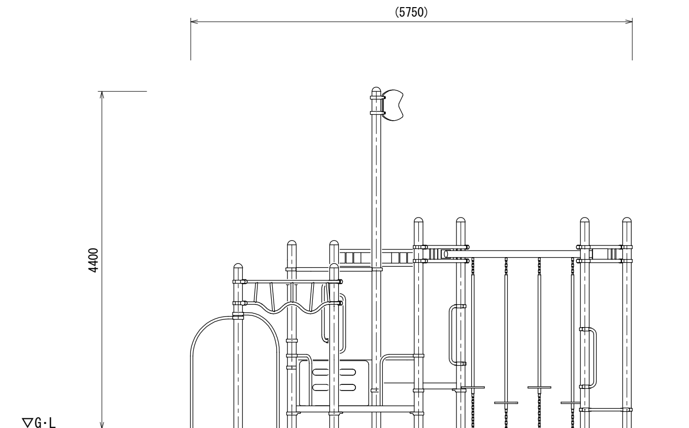
B立面図
