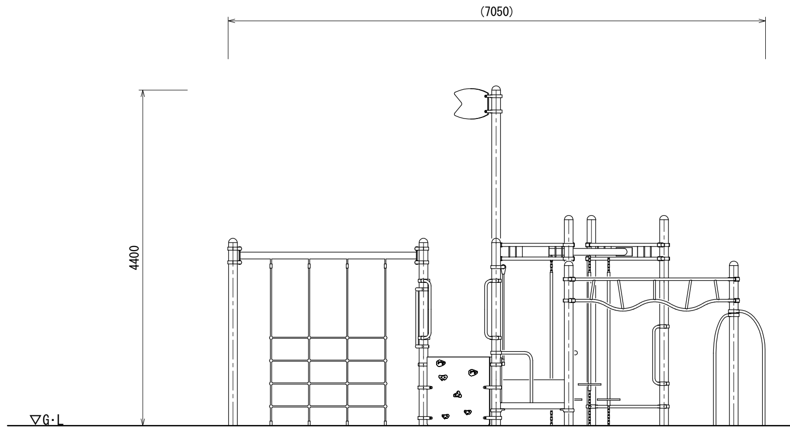
A立面図
