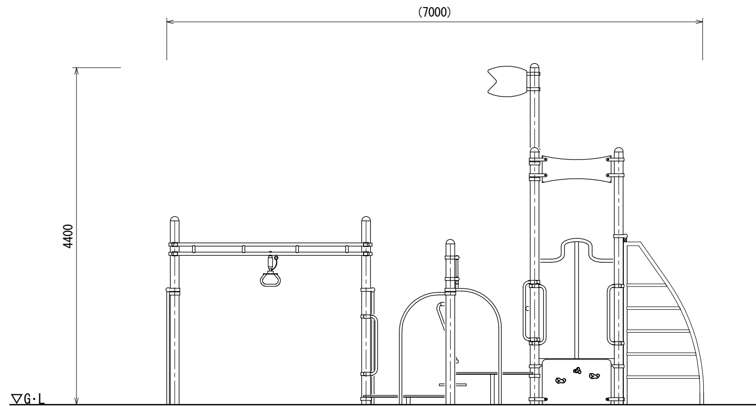
A立面図
