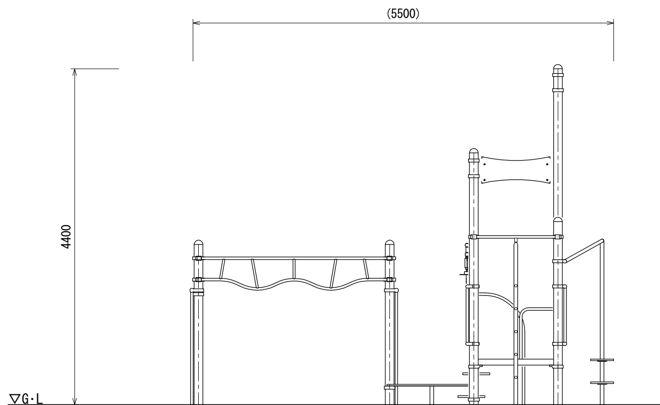
B立面図
