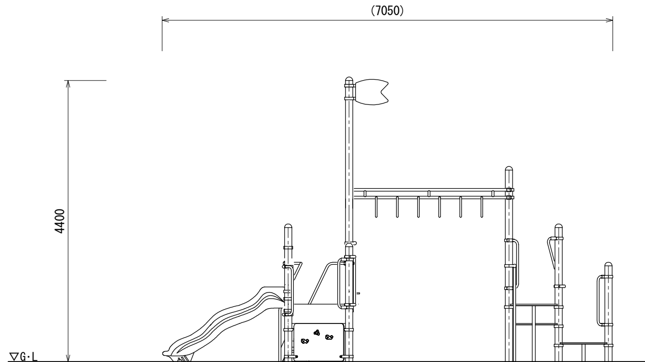
B立面図
