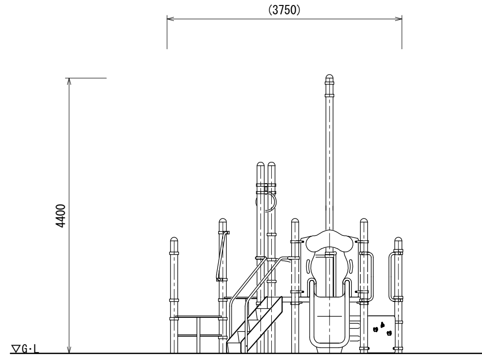
A立面図
