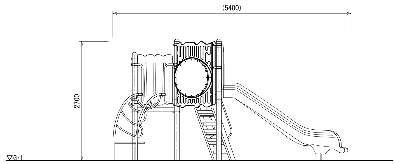
A立面図
