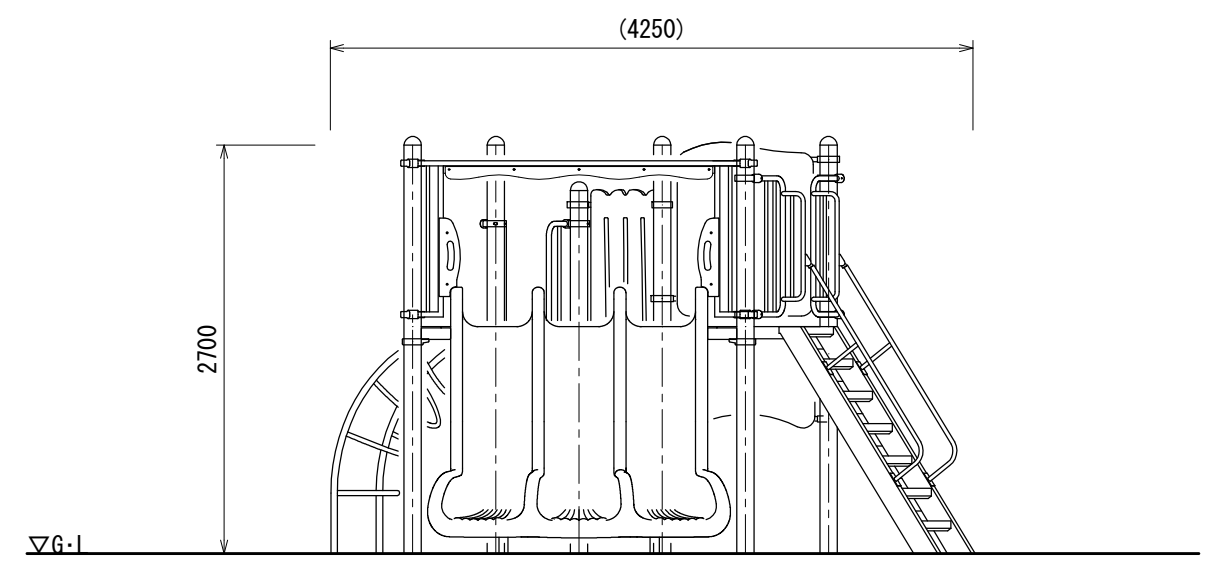
B立面図
