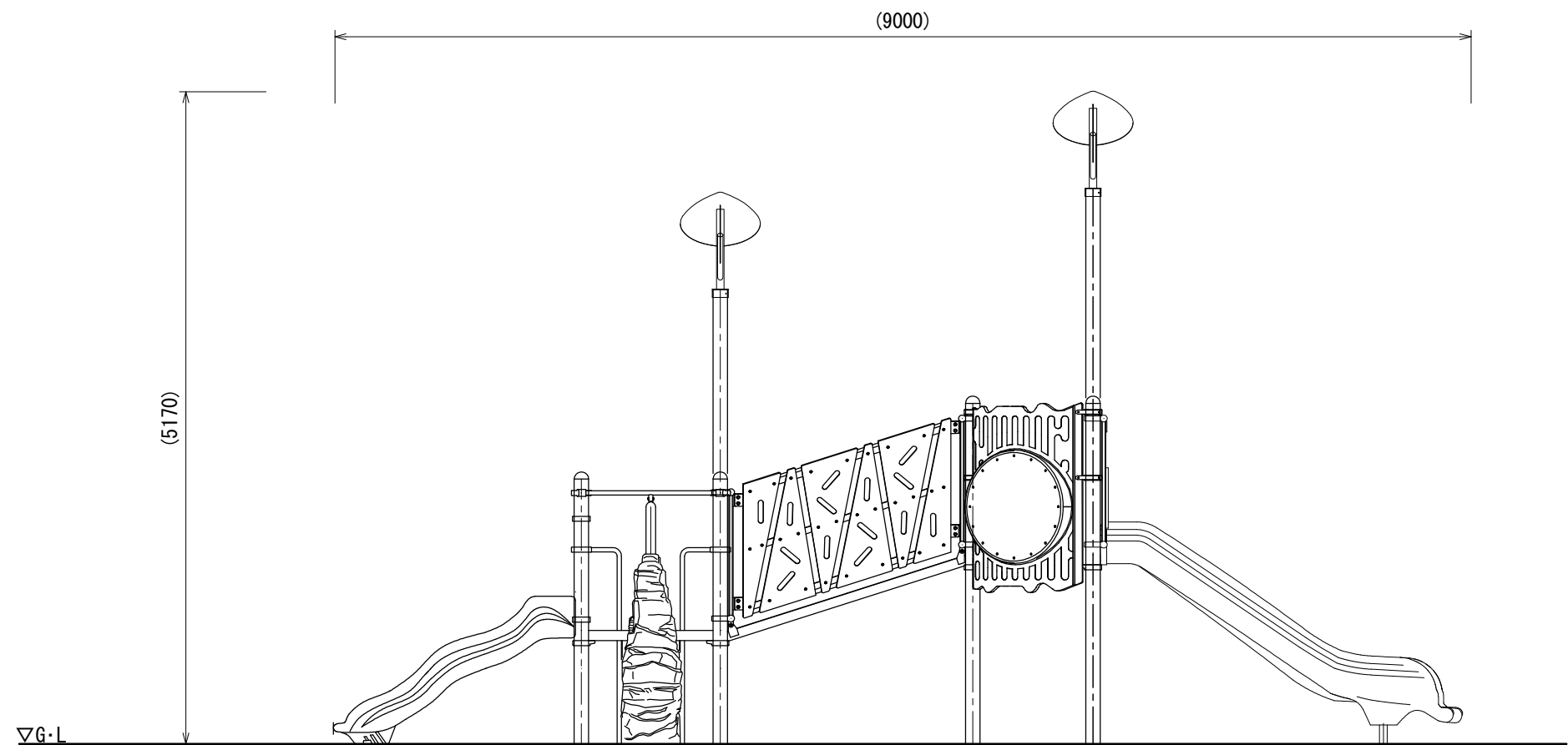
A立面図
