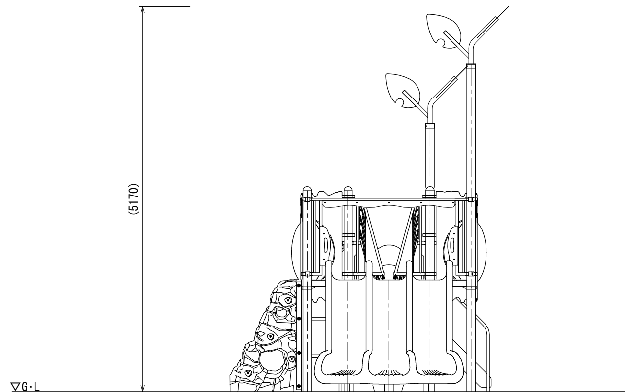
B立面図
