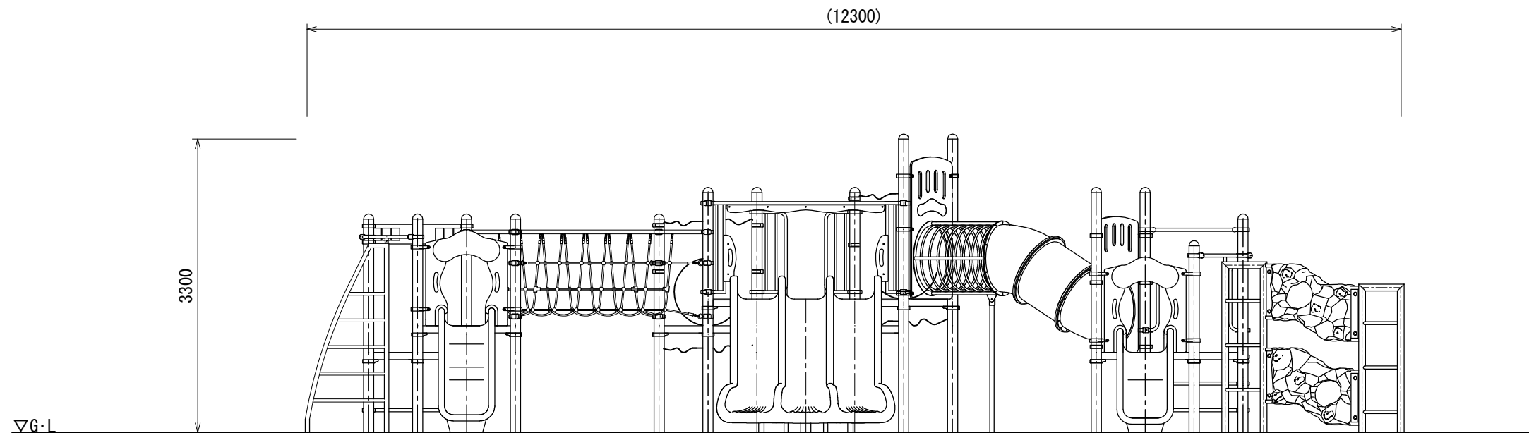
A立面図
