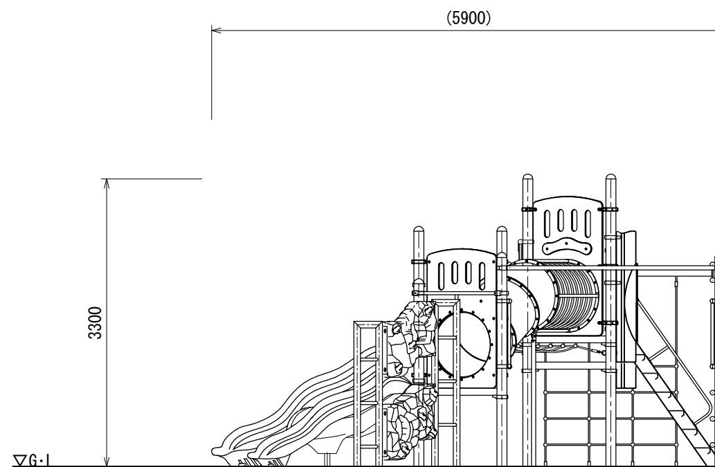
B立面図
