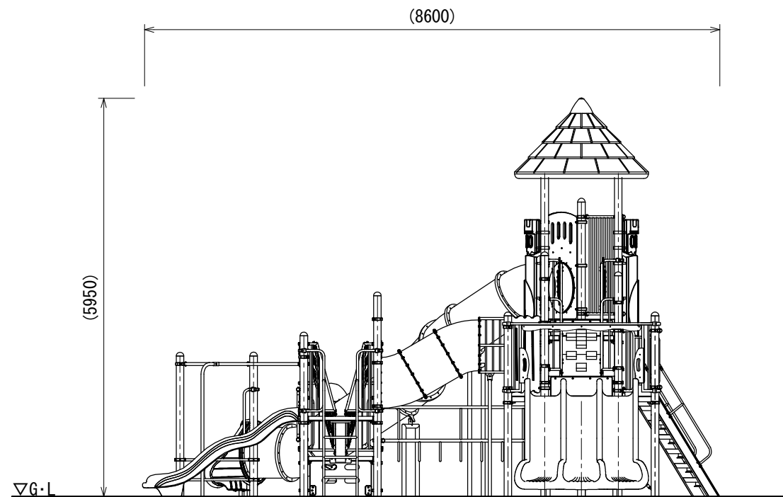
B立面図
