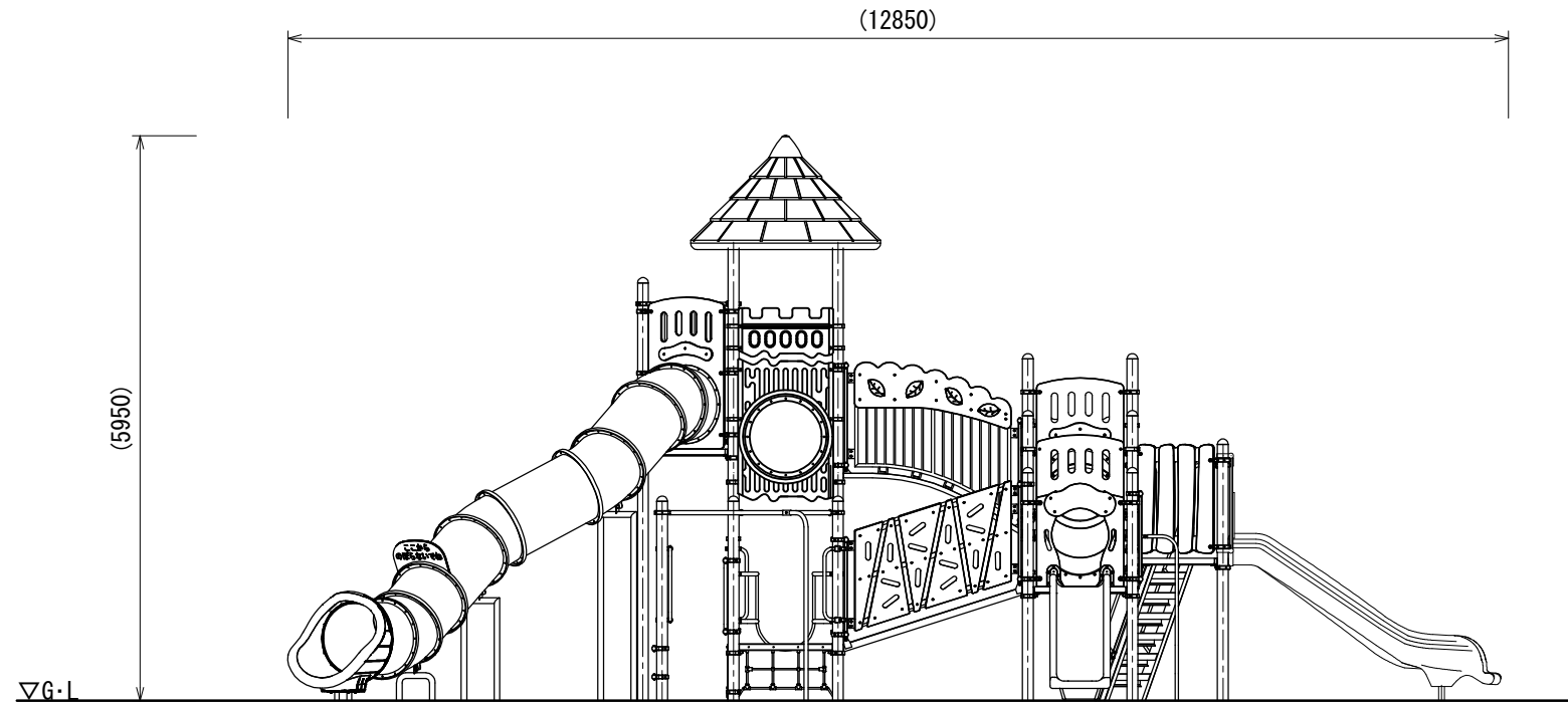
A立面図
