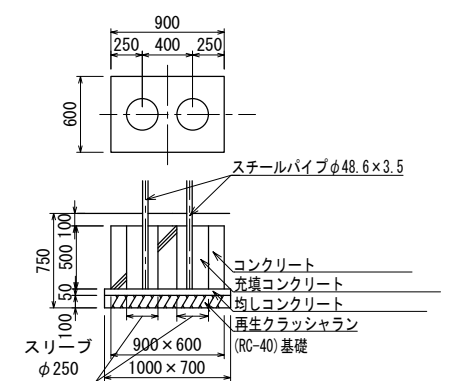
E' 基礎詳細図 (スリーブ穴位置や方向に注意する事)
