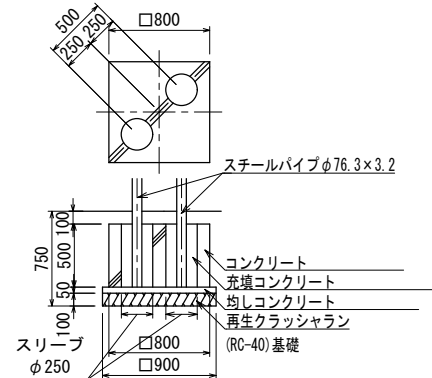
B' 基礎詳細図 (スリーブ穴位置や方向に注意する事)
