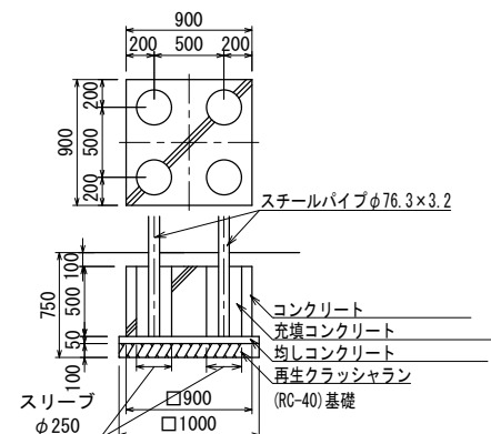
F' 基礎詳細図
