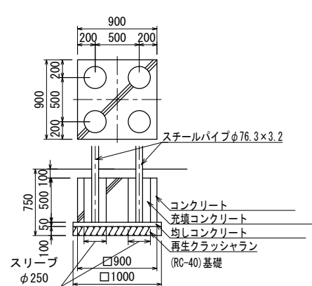
F' 基礎詳細図
