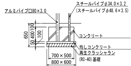
D 基礎詳細図
