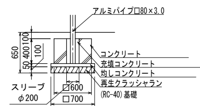
E' 基礎詳細図
