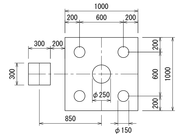
基礎伏図
