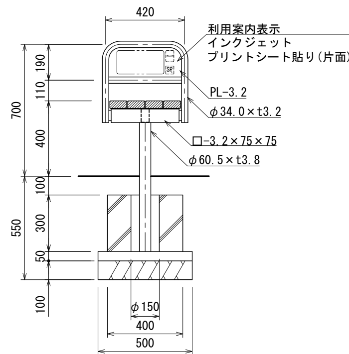
側面図
