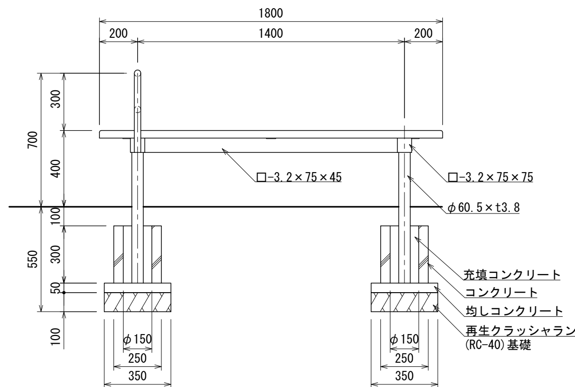
立面図
