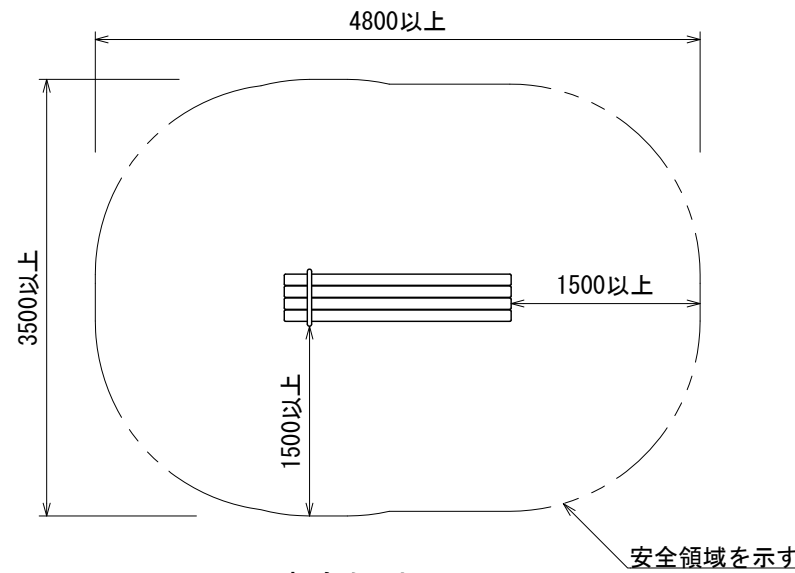
安全領域 S=1:60
