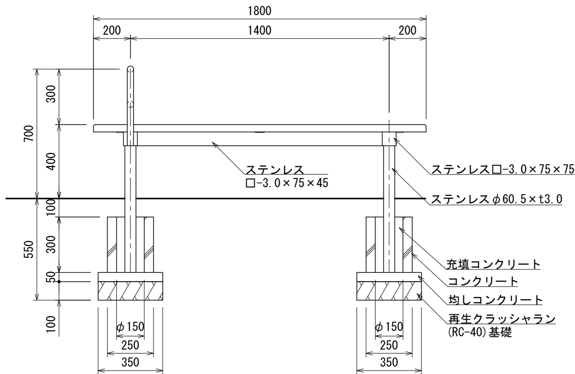
立面図
