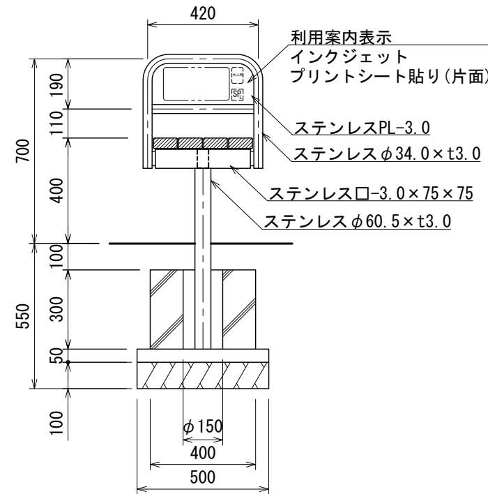
側面図
