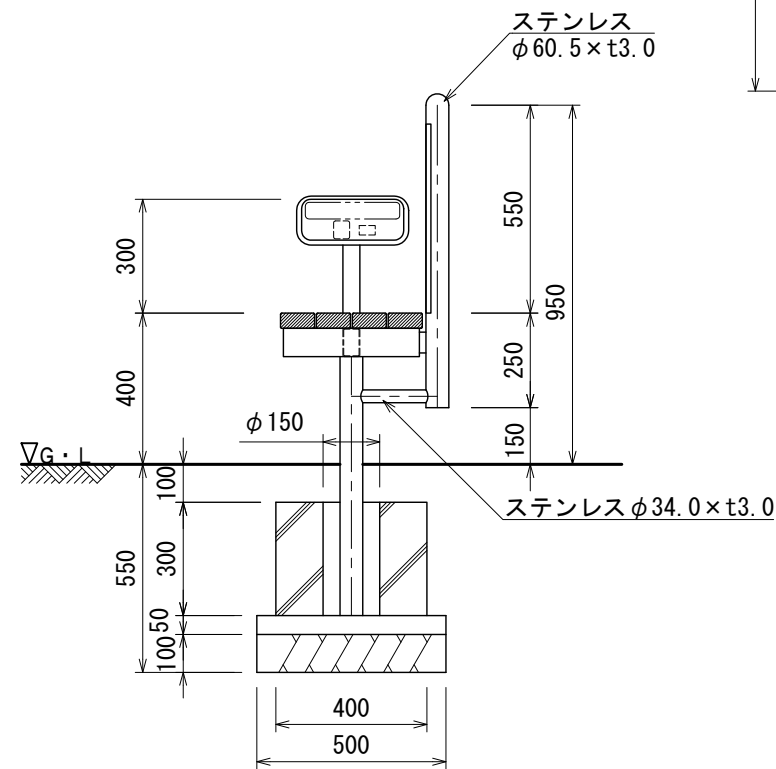
〔座部断面図(2層構造)〕
