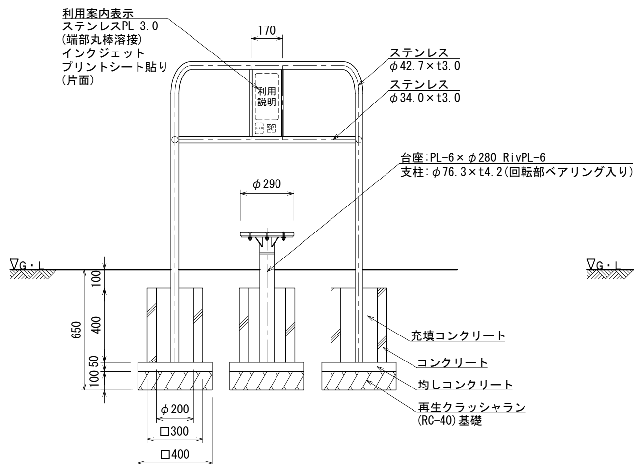
立面図
