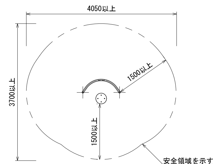
安全領域図 S=1:60
