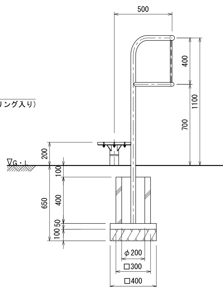
側面図
