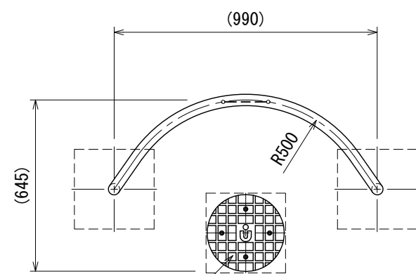
回転ステップ PE積層板 t19 平面図
