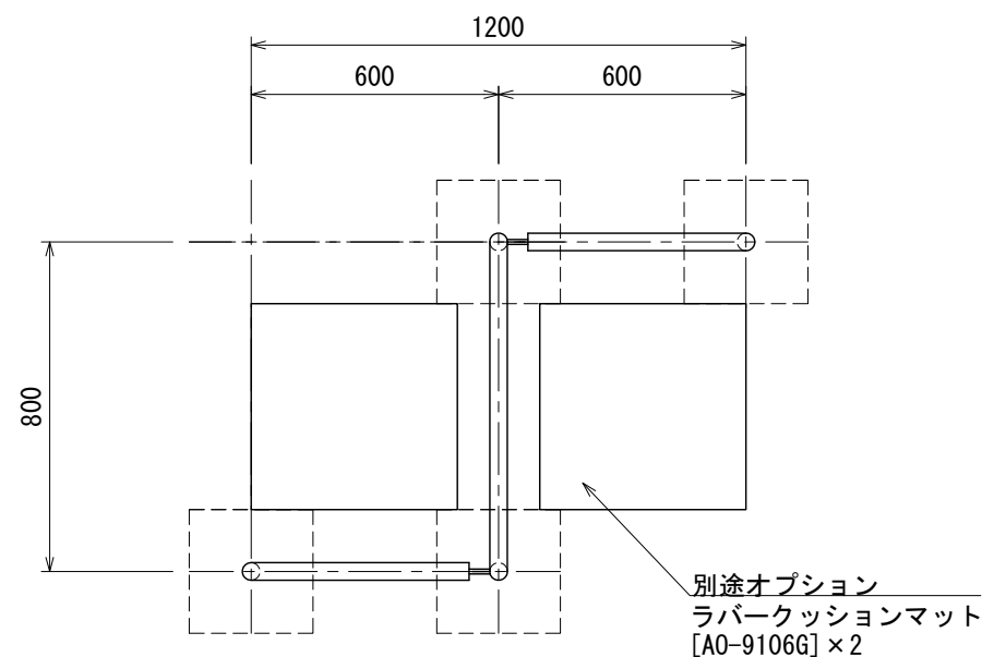
平面図
