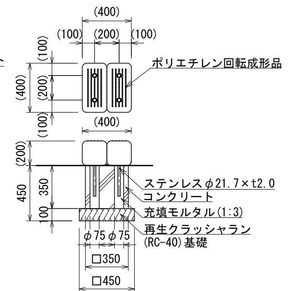
C' 基礎詳細図
