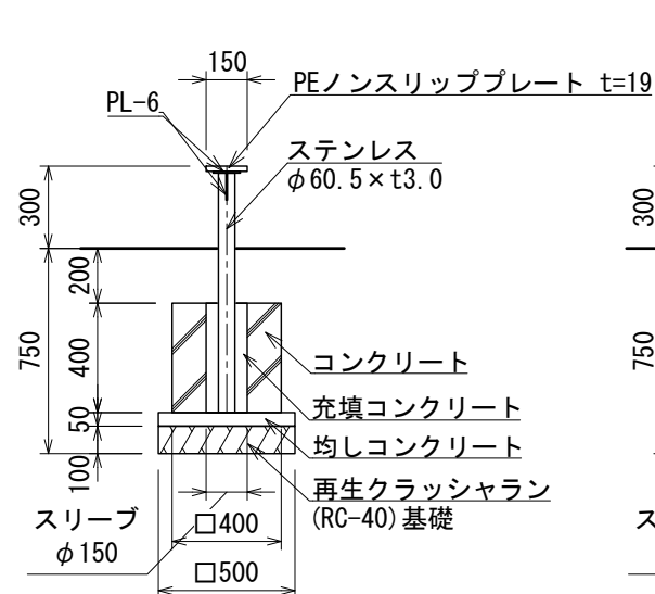
A' 基礎詳細図
