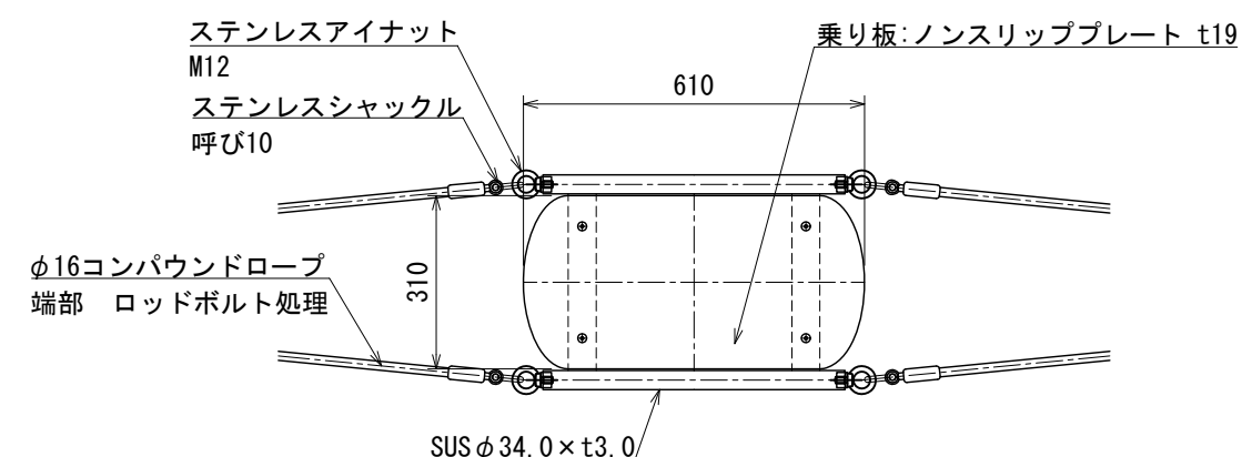
乗り板詳細図 S=1:15
