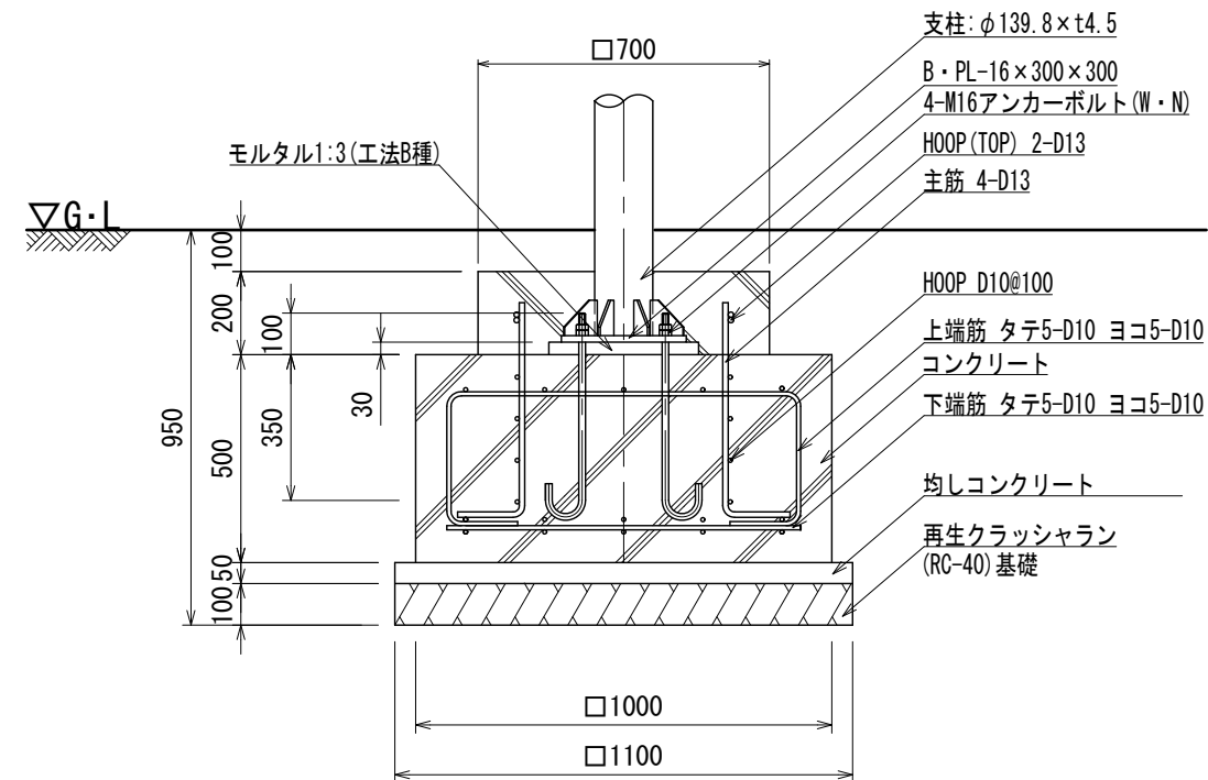
基礎詳細図
