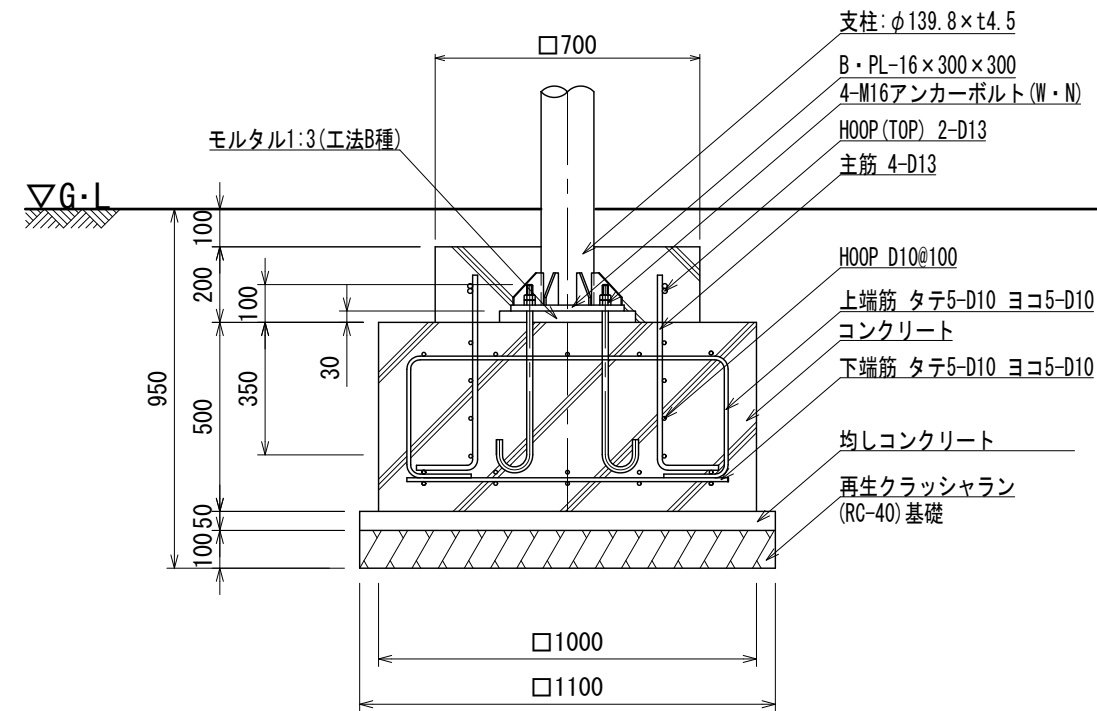
基礎詳細図
