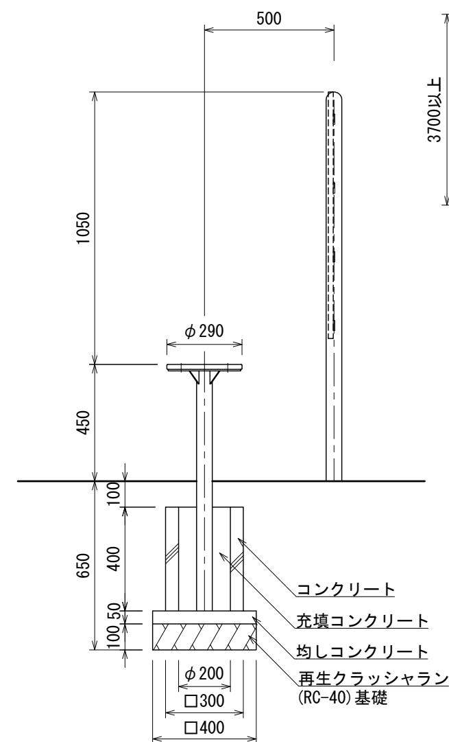
側面図
