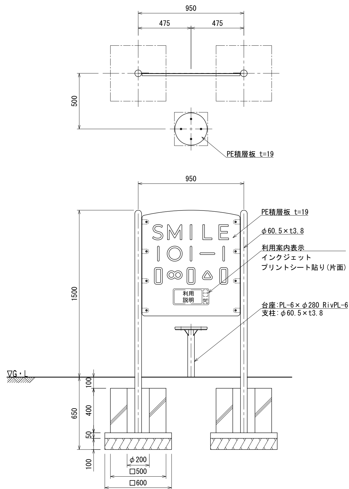
立面図
