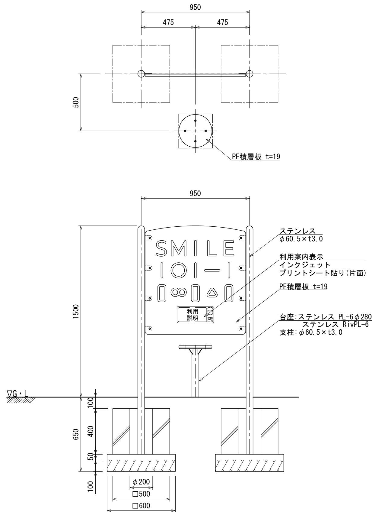
立面図
