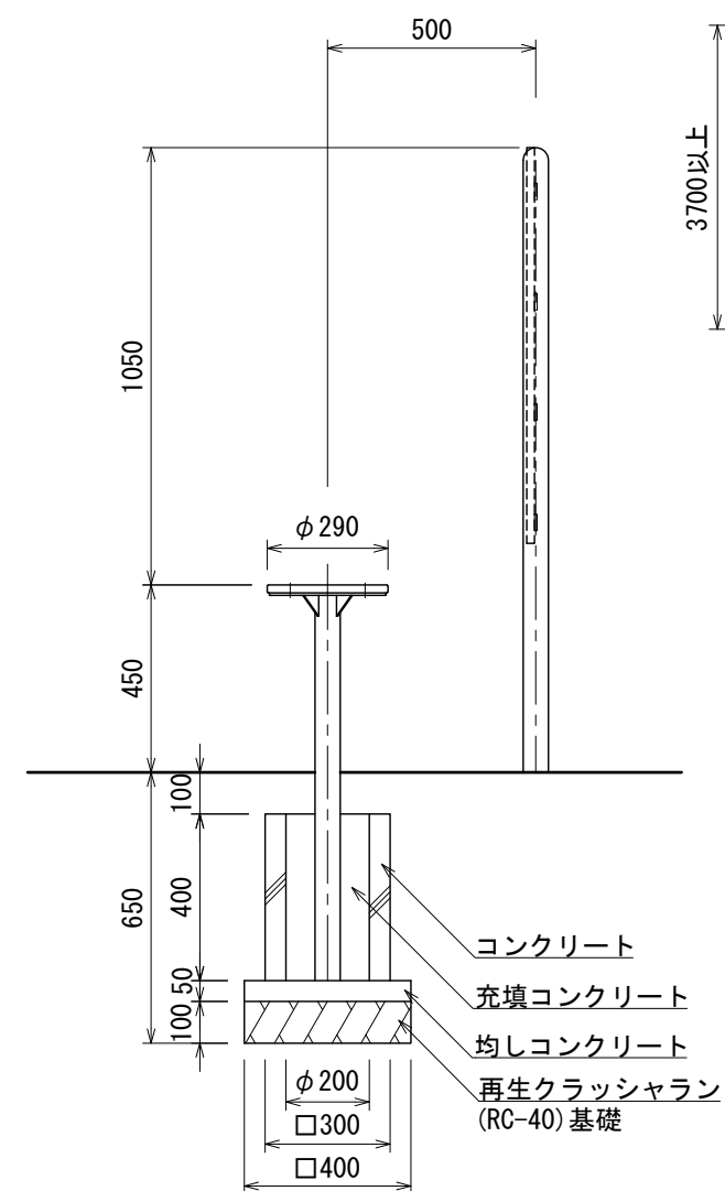
側面図
