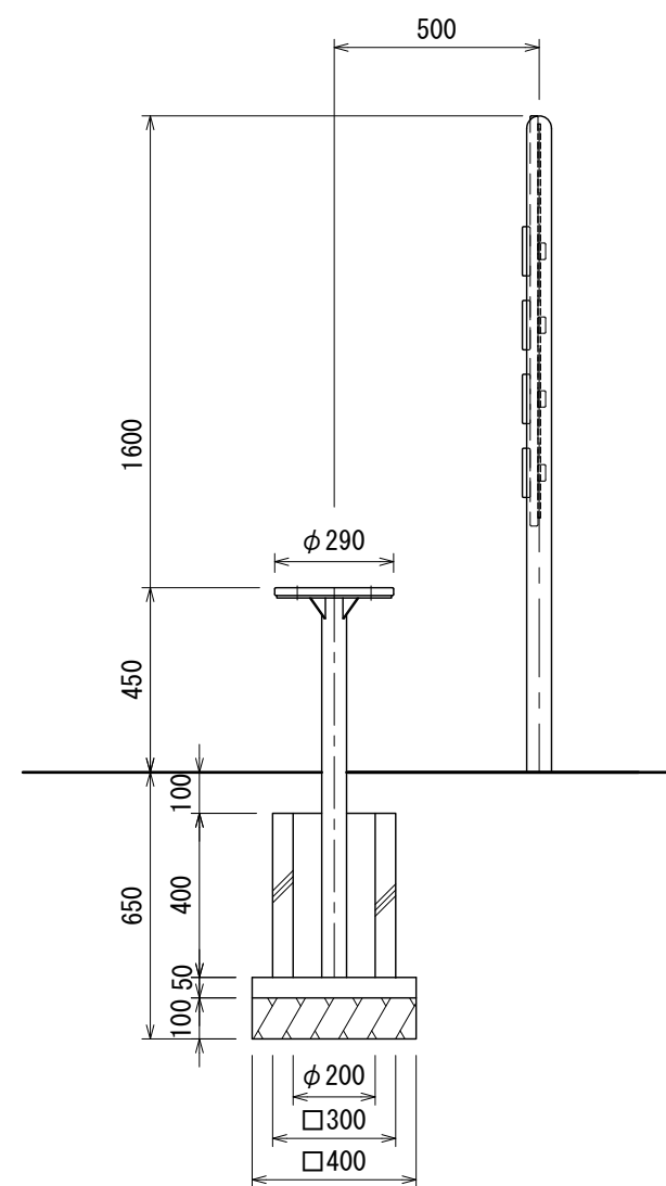
側面図
