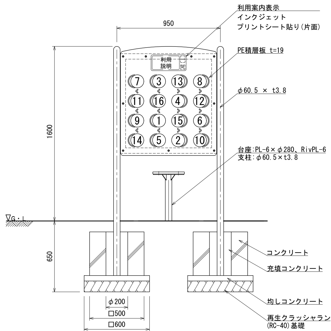
立面図
